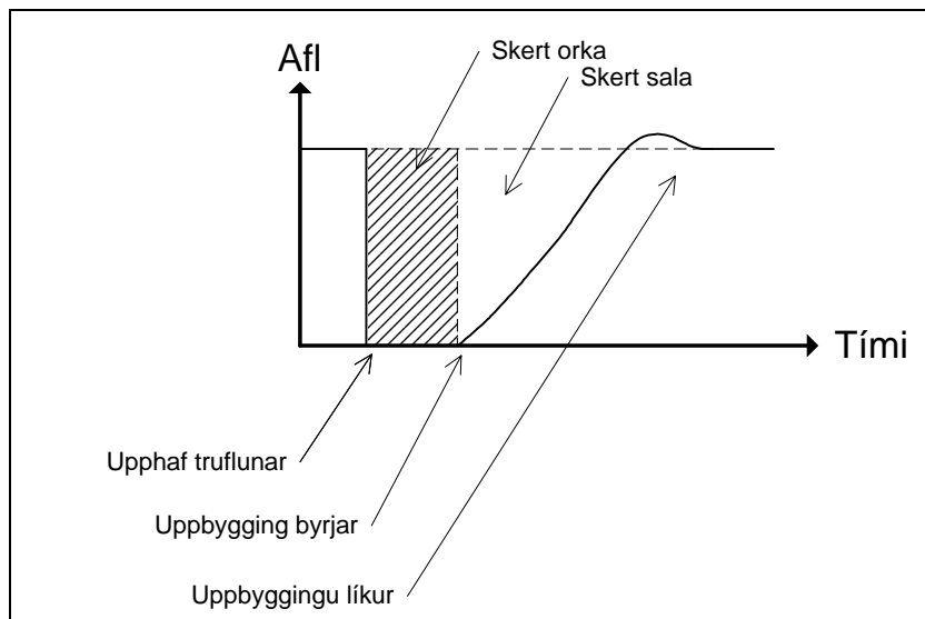
Mynd 12 Dæmi um skerðingu til iðnaðarnotanda.
