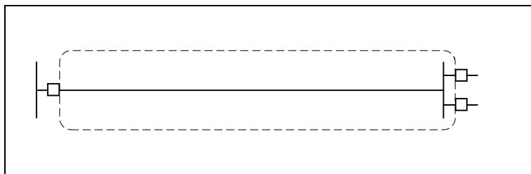
Mynd 5 Kerfiseining þar sem vantar aflrofa fyrir safntein og því er raflínan og safnteinninn ein kerfiseining sem flokkast sem raflína.
