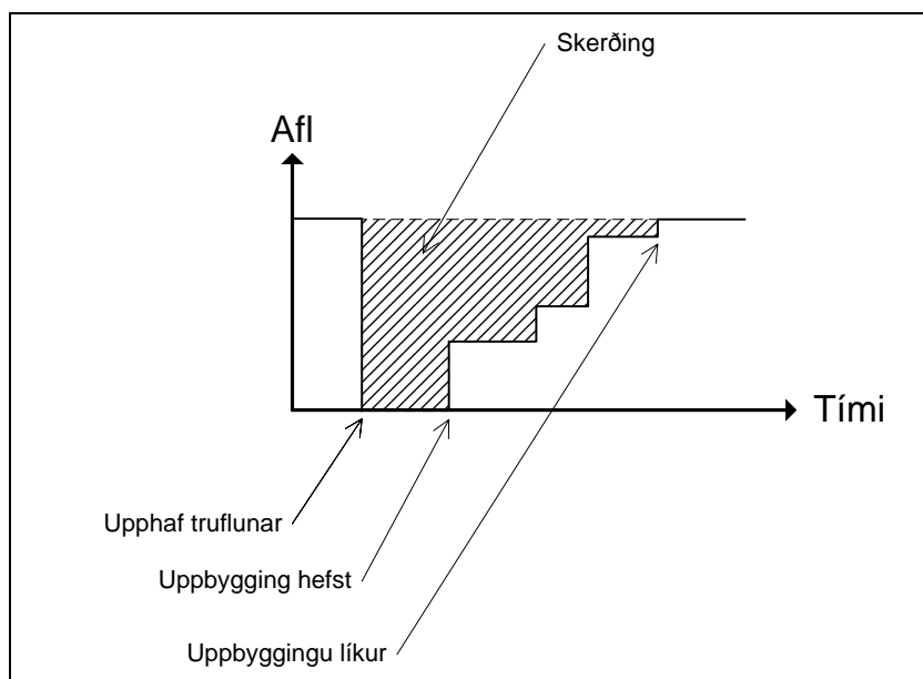
Mynd 13 Dæmi um skerðingu til nokkurra viðskiptavina.
