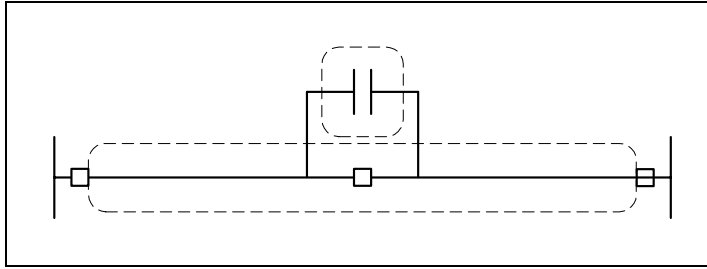
Mynd 6 Tvær kerfiseiningar sem takmarkast af aflrofum. Hér er einungis einn aflrofi sem aðgreinir raðþéttinn og raflínan öll er ein kerfiseining utan þéttisins. Ef raflínan fer út í truflun fer raðþéttirinn einnig út.
