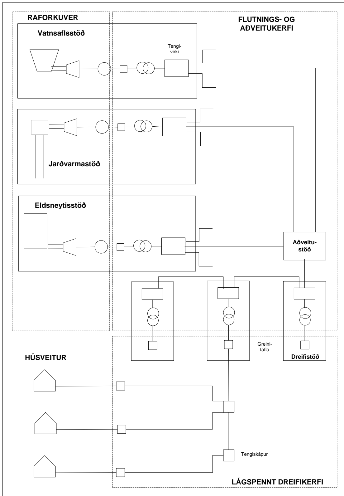
Mynd 1 Skipting raforkukerfisins niður í hluta sem notuð er við skráningu rekstrartruflana.
