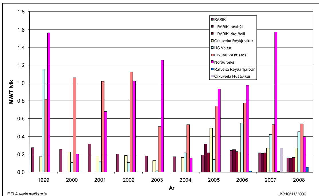
Mynd 4 Stuðull um meðalskerðingu álags, SMA, fyrir aðrar veitur í START hópnum en Landsnet árin 1999-2008.
