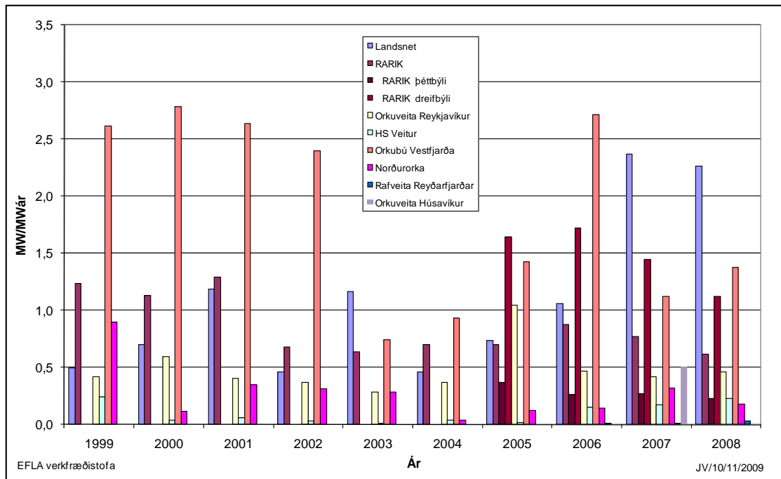
Mynd 1 Stuðull um rofið álag, SRA, fyrir allar veiturnar í START hópnum árin 1999-2008.
