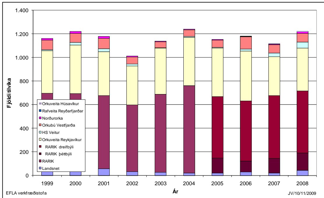
Mynd 7 Fjöldi skerðingartívika árin 1999-2008 sem eru innan við 1 kerfismínúta.
