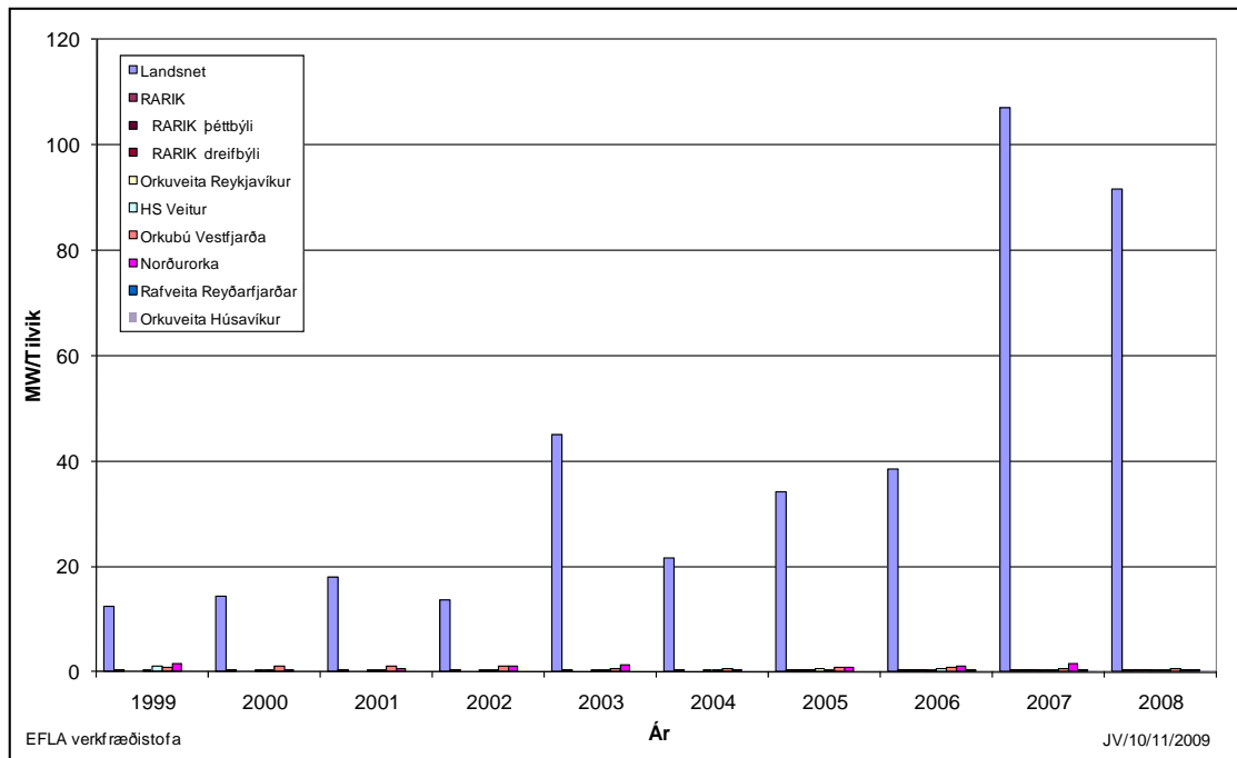
Mynd 3 Stuðull um meðalskerðingu álags, SMA, fyrir allar veiturnar í START hópnum árin 1999-2008.
