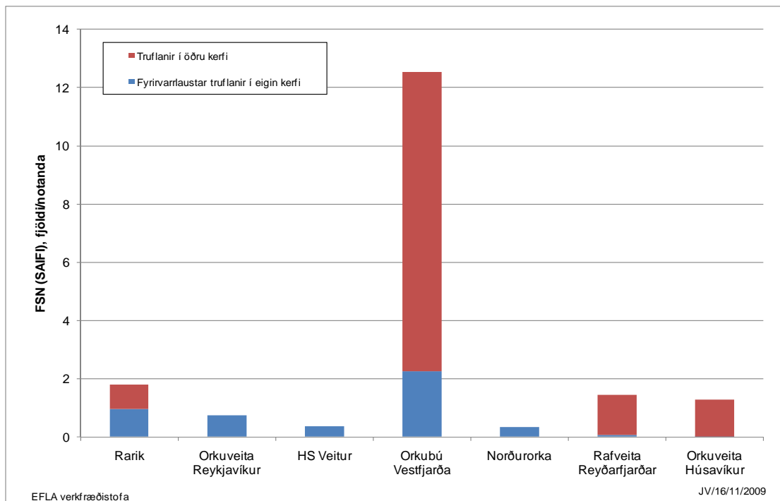
Mynd 19 Stuðull um fjölda straumleysistilvika á hvern notanda, FSN (SAIFI), árið 2008.
