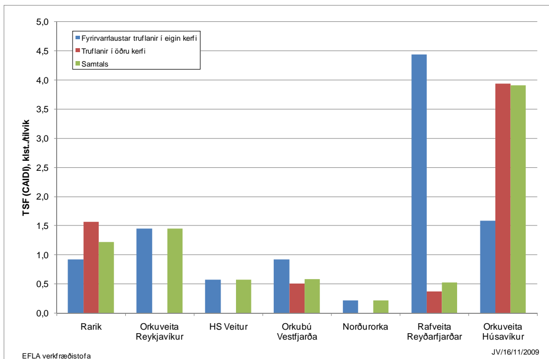
Mynd 21 Stuðull um tímalengd straumleysis á hvert tilvik skerðingar, TFSF (CAIDI), árið 2008 (kst./tilvik).
