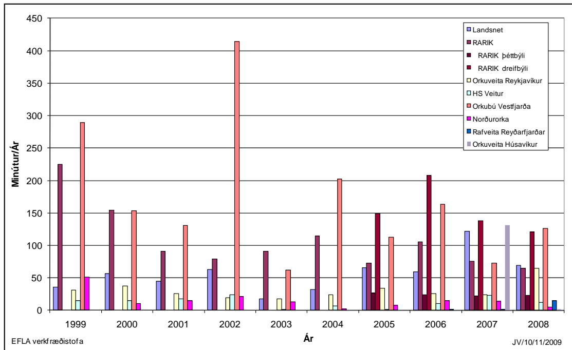
Mynd 5 Stuðull um meðallengd skerðingar, SMS, fyrir allar veiturnar í START hópnum árin 1999-2008.
