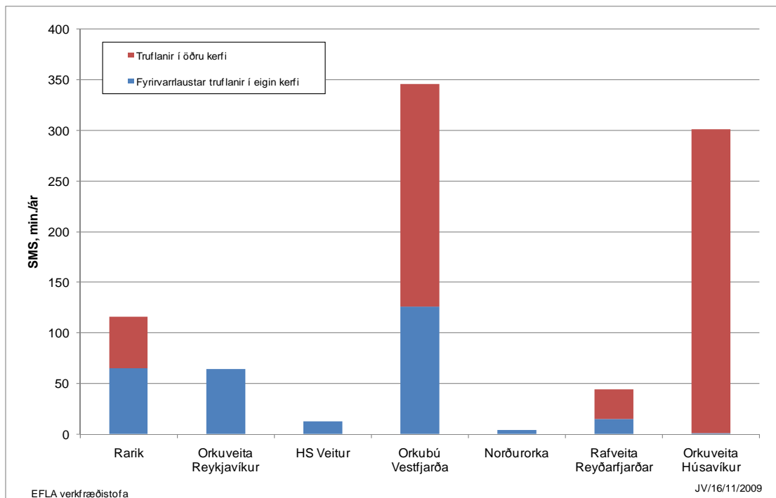
Mynd 17 Stuðull um meðallengd skerðingar, SMS, fyrir allar veiturnar í START hópnum árið 2008.
