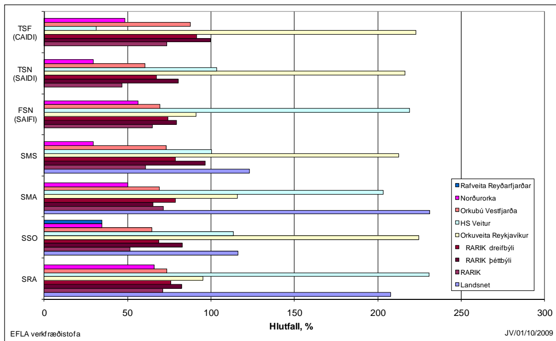
Mynd I Samanburður á truflunum í raforkukerfi Landsnets og stærstu dreifiveitnanna árið 2008 við meðaltal árána 1999-2008 (árið 2008 í hlutfalli við meðaltalið).
