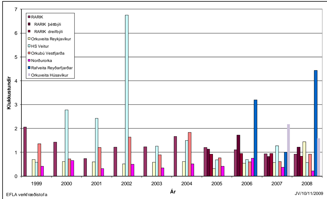
Mynd 13 Stuðull um tímalengd straumleysis á hvert tilvik skerðingar, TSF (CAIDI), árin 1999-2008 (klst/tilvik).
