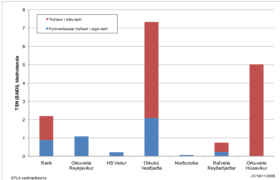
Mynd 20 Stuðull um tímalengd straumleysis á hvern notanda, TSN (SAIDI), árið 2008.
