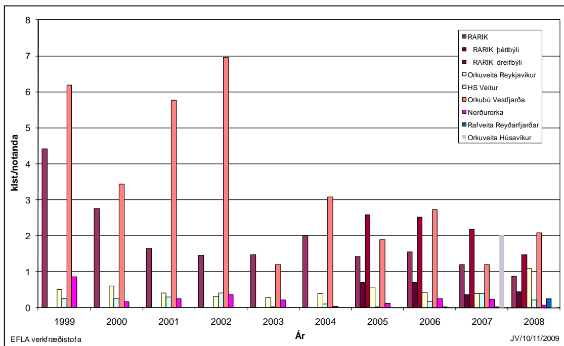
Mynd 12 Stuðull um tímalengd straumleysis á hvern notanda, TSN (SAIDI), árin 1999-2008.
