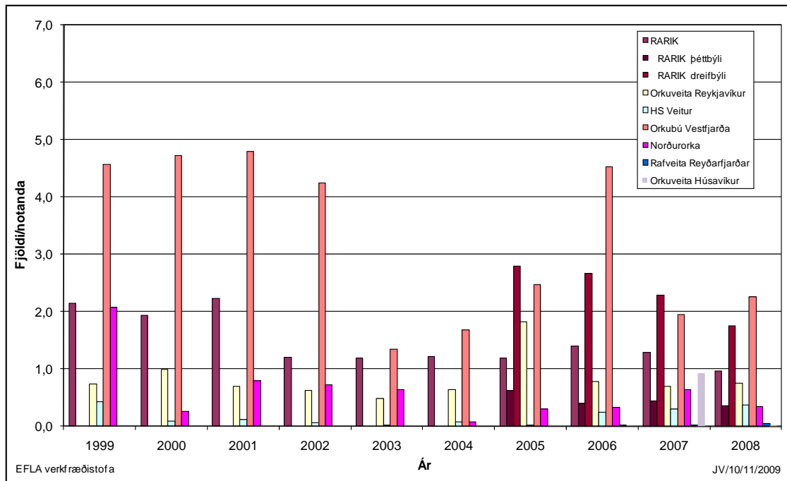
Mynd 11 Stuðull um fjölda straumleysistilvika á hvern notanda, FSN (SAIFI), árin 1999-2008.
