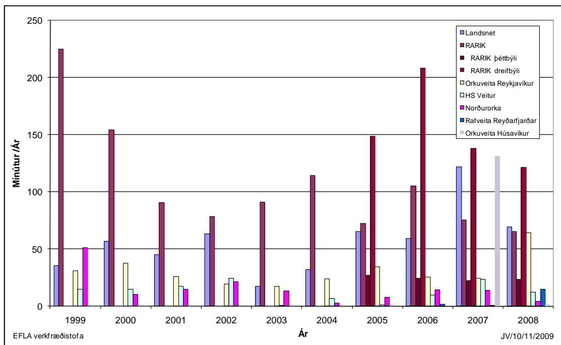
Mynd 6 Stuðull um meðallengd skerðingar, SMS, fyrir aðrar veitur í START hópnum en Orkubú Vestfjarða árin 1999-2008.
