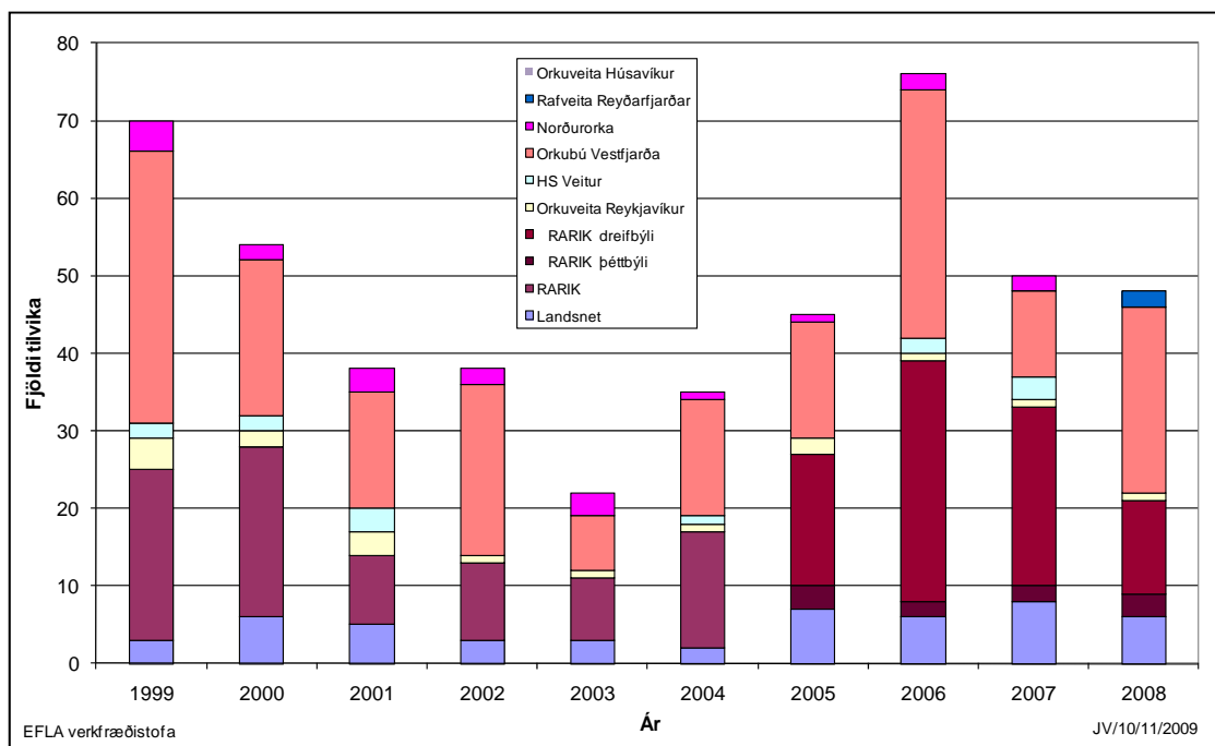
Mynd 8 Fjöldi skerðingartívika árin 1999-2008 sem eru á bilinu 1 til 10 kerfismínútur.
