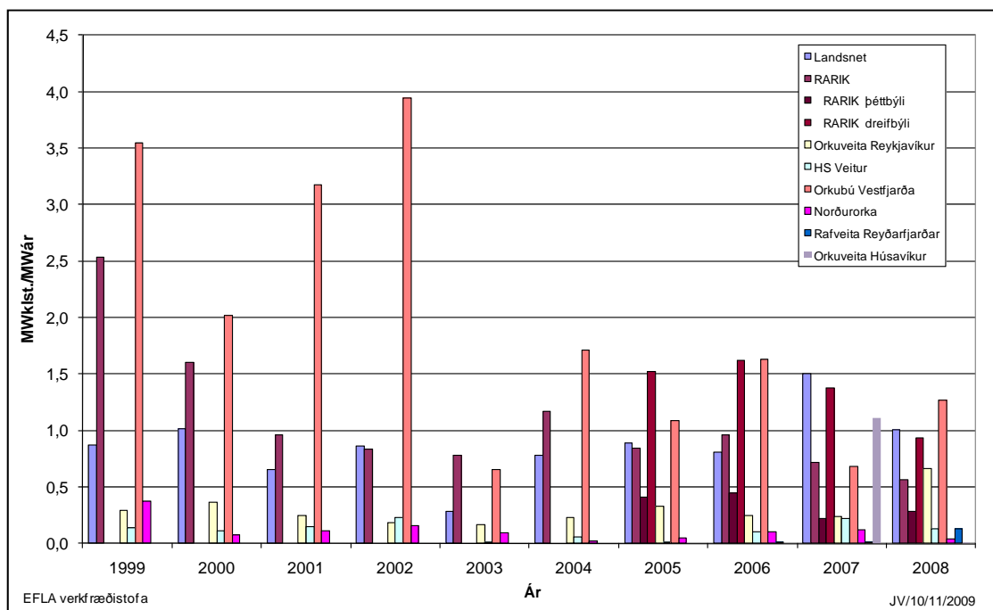
Mynd 2 Stuðull um skerta orkuafhendingu, SSO, fyrir allar veiturnar í START hópnum árin 1999-2008.
