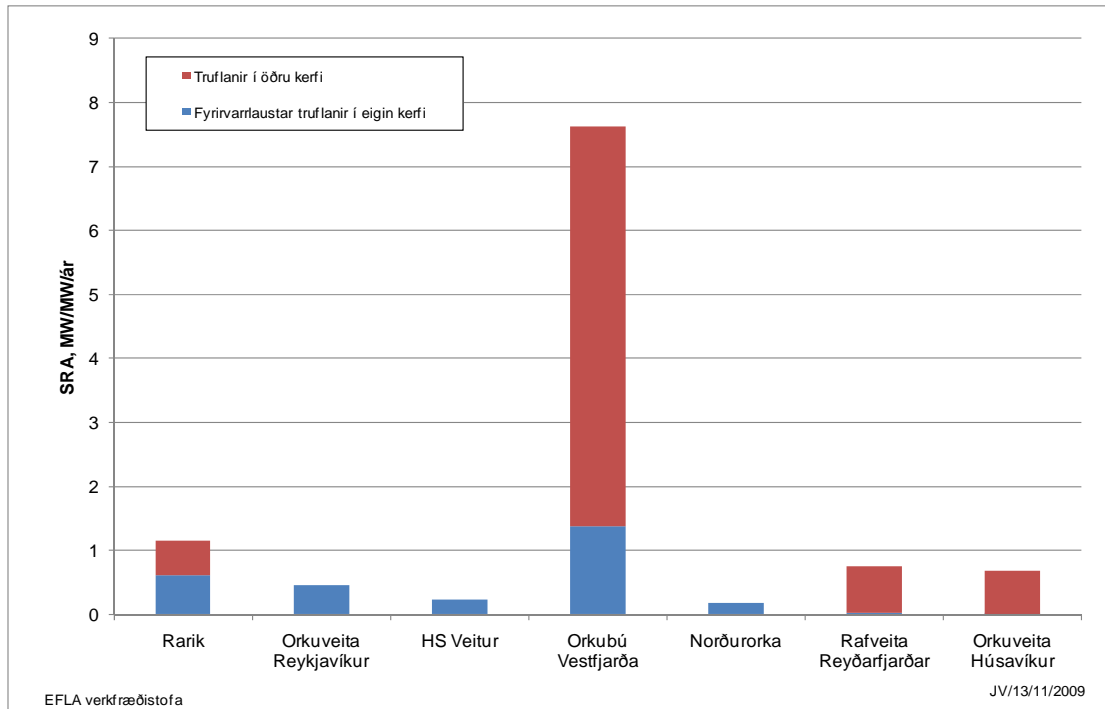
Mynd 14 Stuðull um rofið álag, SRA, fyrir allar veiturnar í START hópnunum árið 2008.
