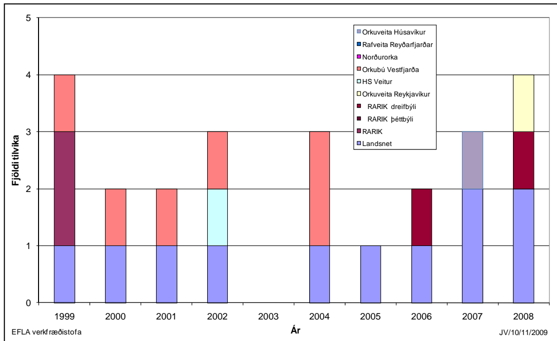
Mynd 9 Fjöldi skerðingartilvika árin 1999-2008 sem eru á bilinu 10 til 100 kerfismínútur.
