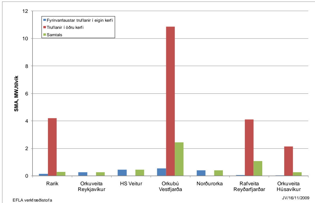
Mynd 16 Stuðull um meðalskerðingu álags, SMA, fyrir allar veiturnar í START hópnum árið 2008.
