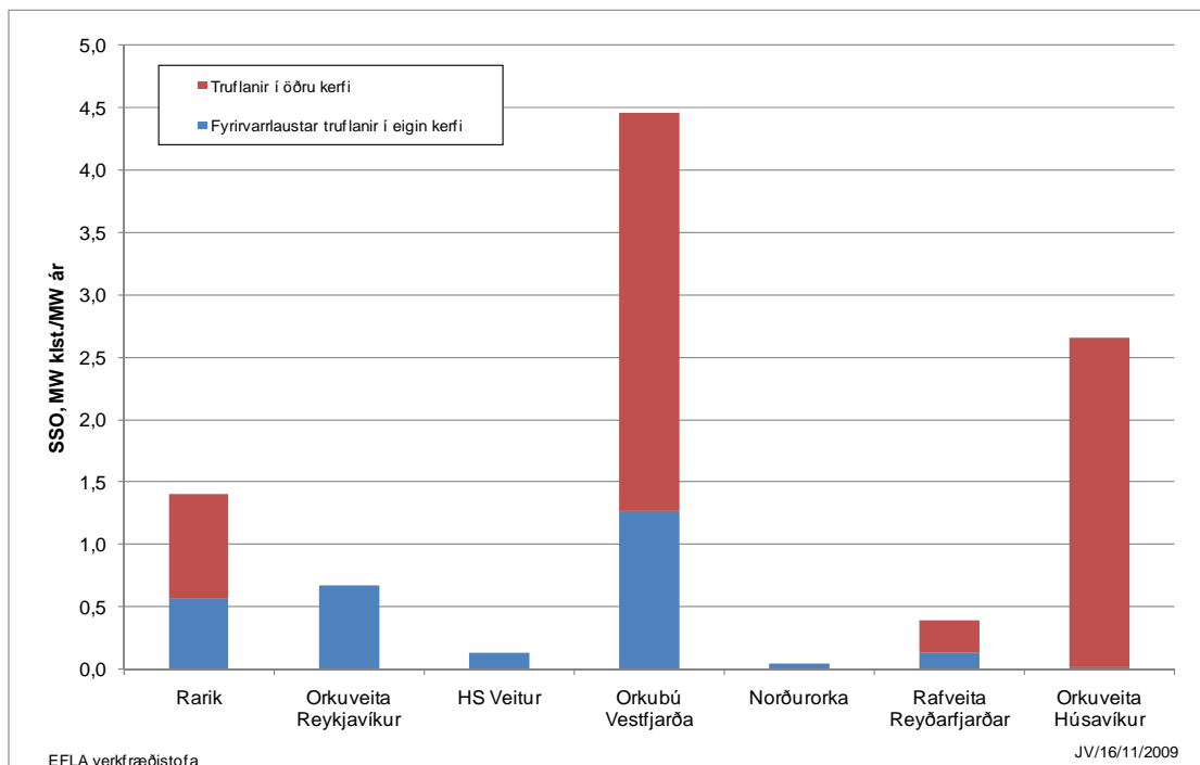
Mynd 15 Stuðull um skerta orkuafhendingu, SSO, fyrir allar veiturnar í START hópnunum árið 2008.
