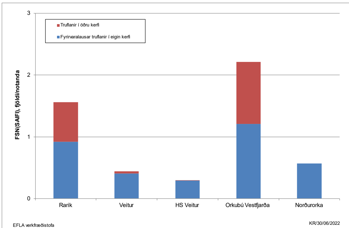
MYND 34 Stuðull um fjölda straumleysistilvika á hvern notanda, FSN (SAIFI), árið 2021 (fjöldi/notanda).
