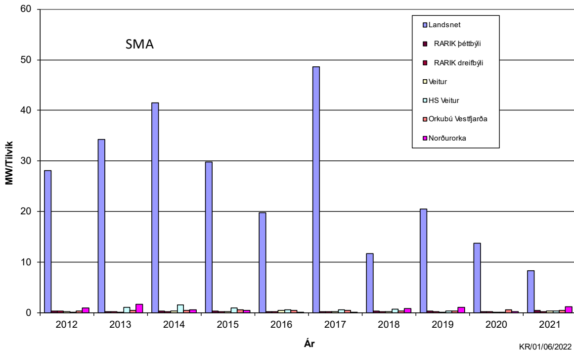
MYND 4 Stuðull um meðalskerðingu álags, SMA, fyrir árin 2012-2021
