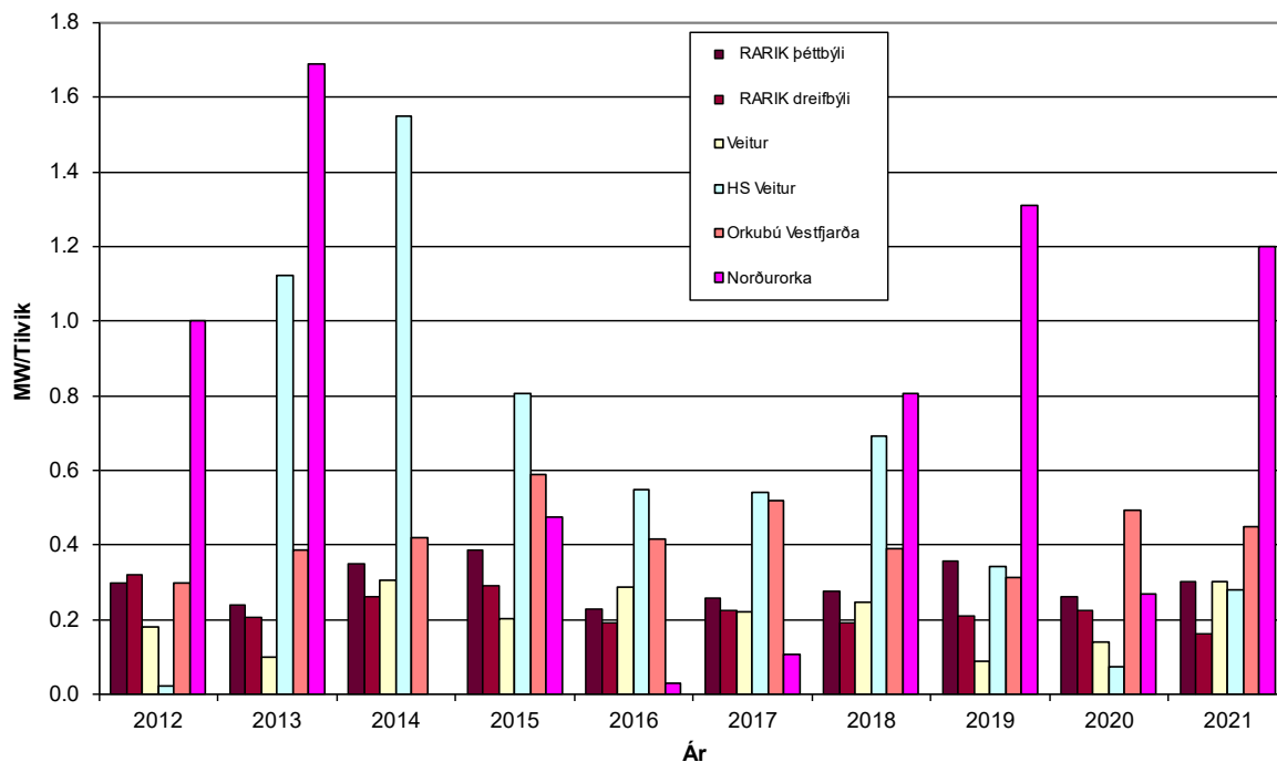
MYND 23 Stuðull um meðalskerðingu álags, SMA, fyrir aðrar veitur en Landsnet, fyrir truflanir sem vara lengur en 3 mínútur árin 2012-2021.
