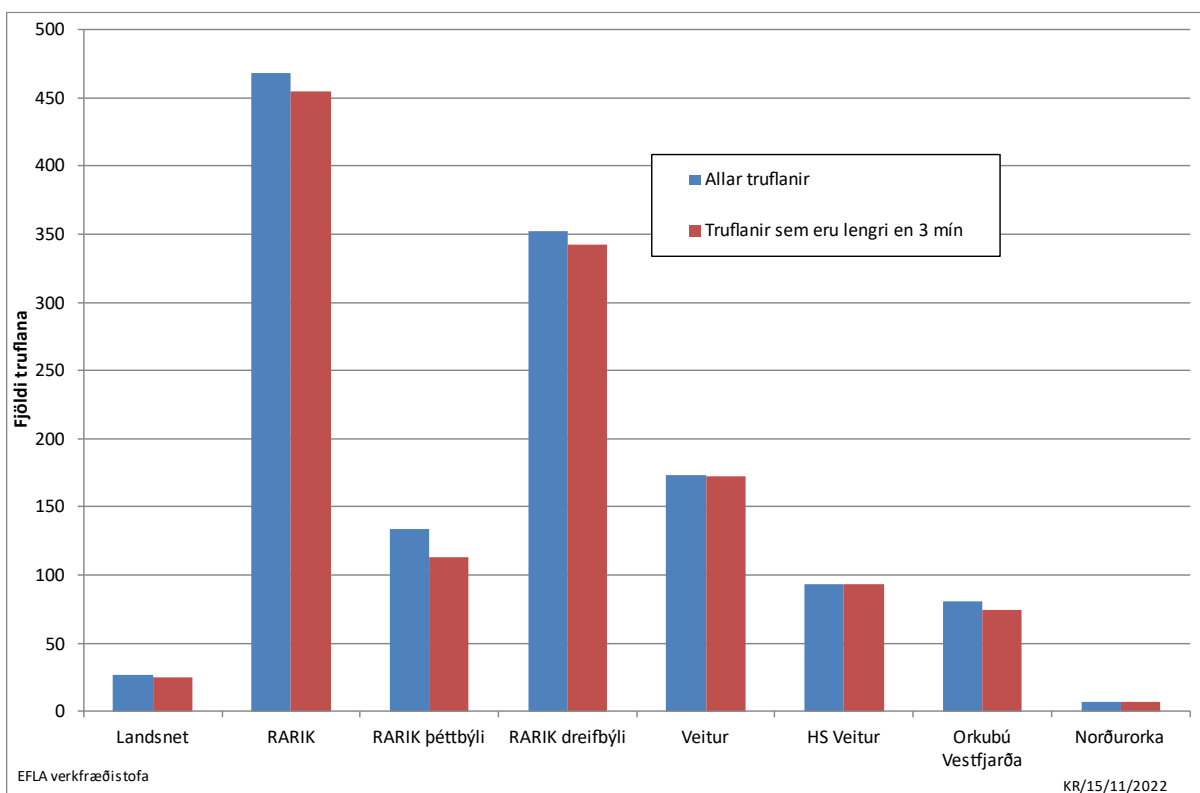
MYND 16 Heildarfjöldi skerðingartilvika árið 2021, sýndar eru annars vegar allar truflanir og hins vegar truflanir sem vara lengur en 3 mínútur.
