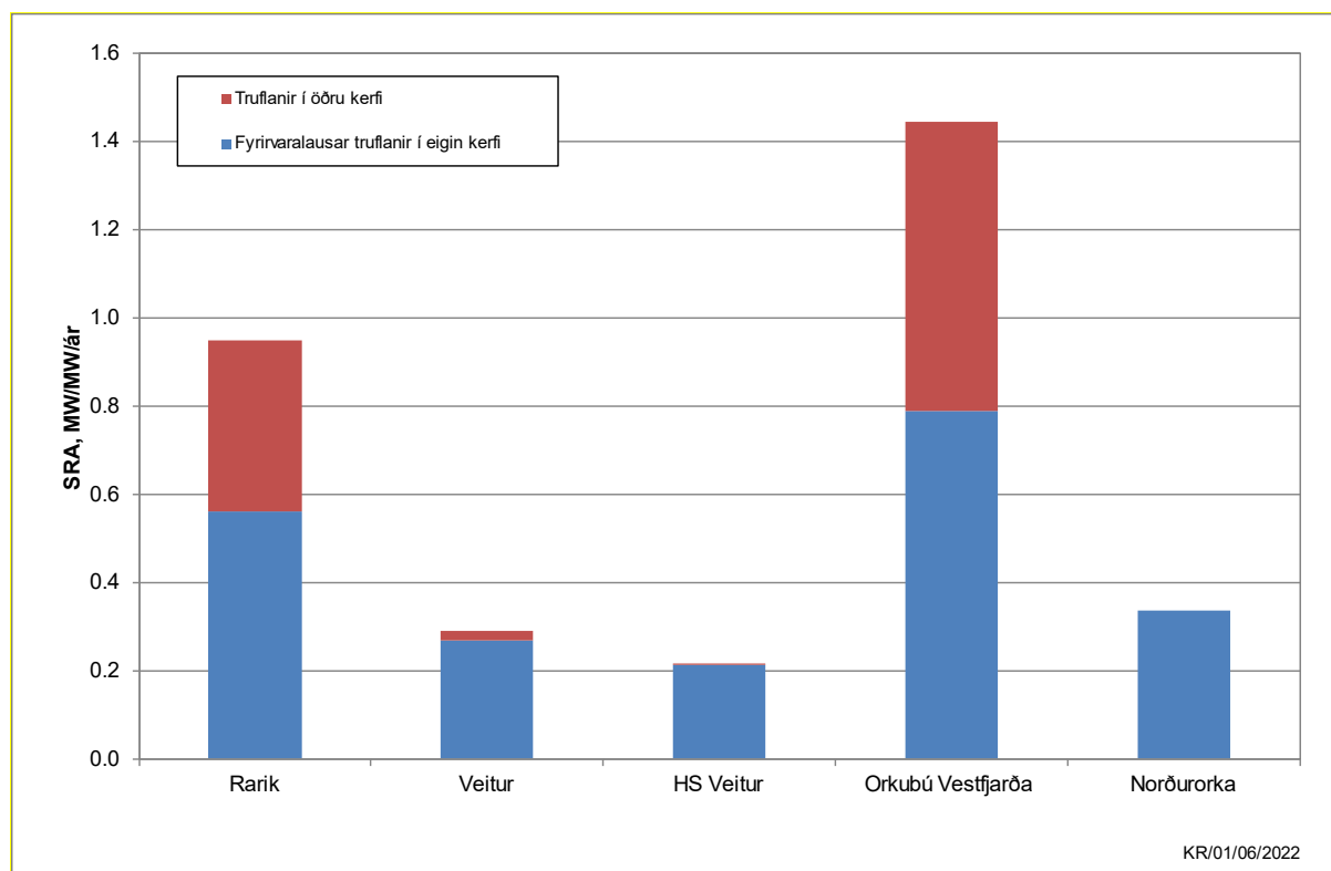
MYND 30 Stuðull um rofið álag, SRA, árið 2021.
