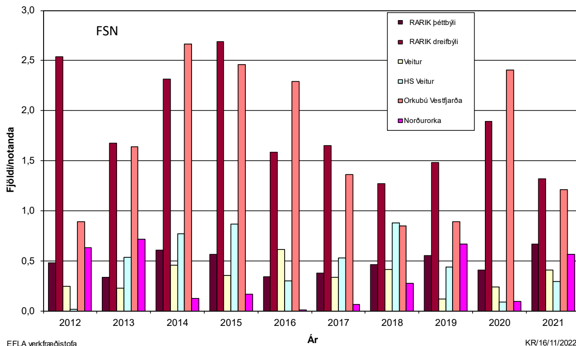
MYND 11 Stuðull um fjölda straumleysistilvika á hvern notanda, FSN (SAIFI), árin 2012-2021.
