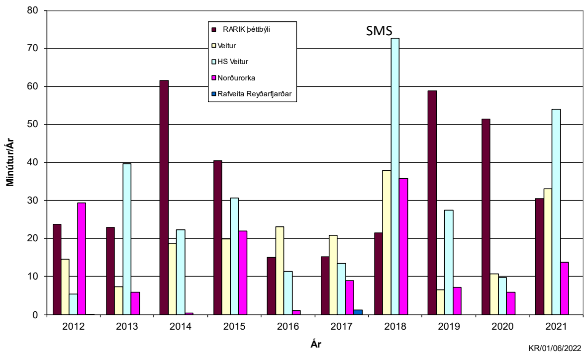
MYND 7 Stuðull um meðallengd skerðingar, oft nefnt straumleysismínútur, SMS, fyrir aðrar veitur en Orkubú Vestfjarða, RARIK dreifbýli og Landsnet, fyrir árin 2012-2021
