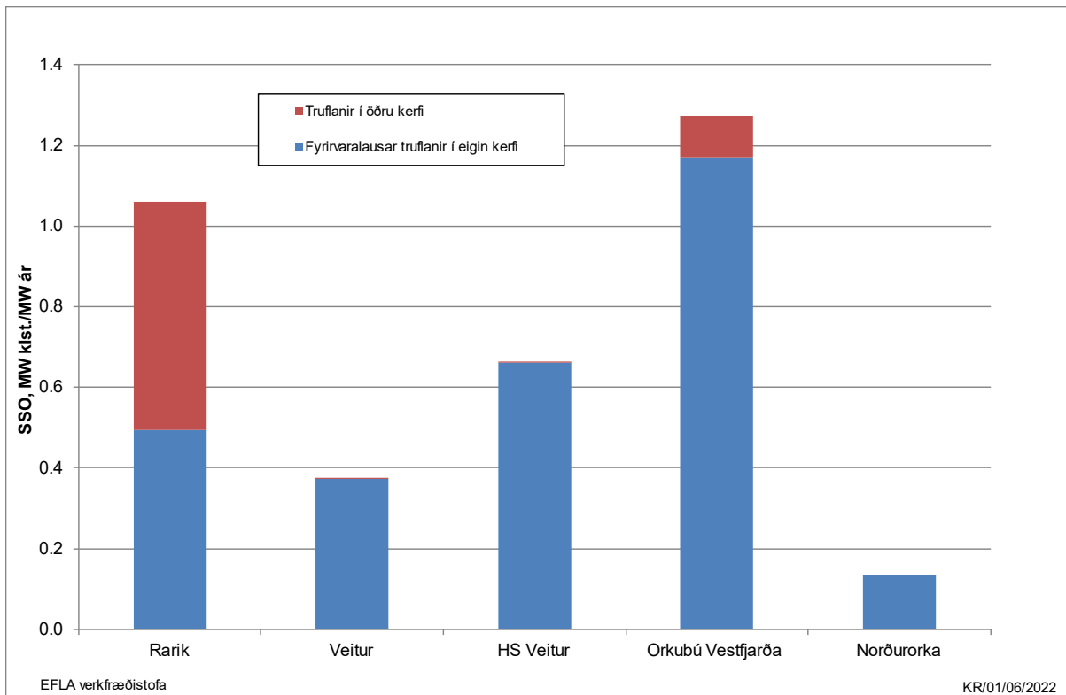
MYND 31 Stuðull um skerta orkuafhendingu, SSO árið 2021.
