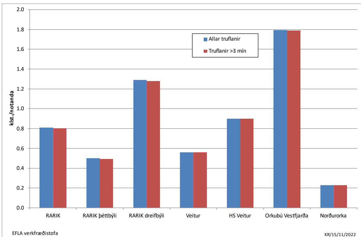
MYND 18 Stuðull um tímalengd straumleysis á hvern notanda, TSN (SAIDI), árið 2021, fyrir allar truflanir og truflanir sem vara lengur en 3 mínútur.
