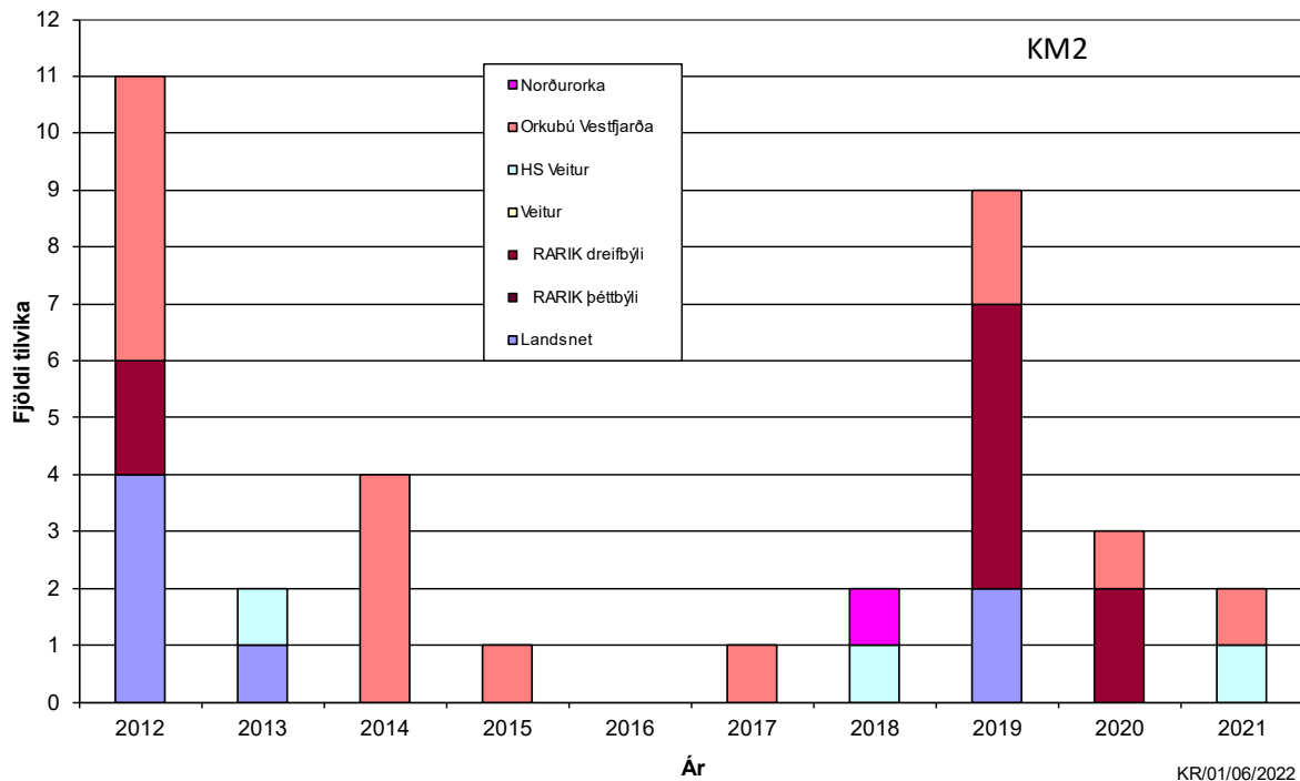
MYND 10 Fjöldi skerðingartilvika árin 2012-2021 sem eru á bilinu 10 til 100 kerfismínútur.
