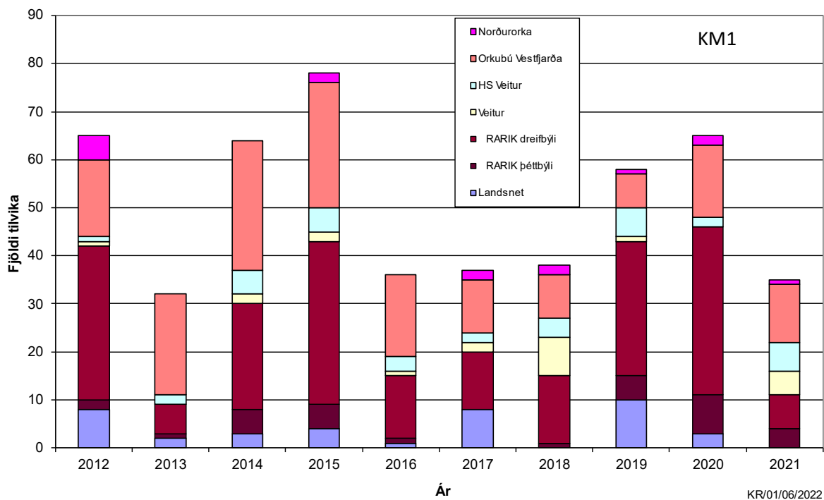
MYND 9 Fjöldi skerðingartilvika árin 2012-2021 sem eru á bilinu 1 til 10 kerfismínútur.
