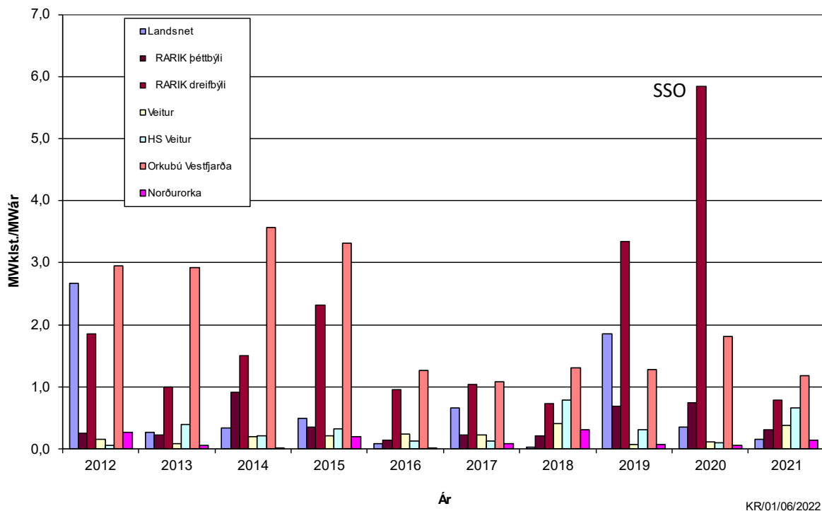
MYND 3 Stuðull um skerta orkuafhendingu, SSO, fyrir árin 2012-2021
