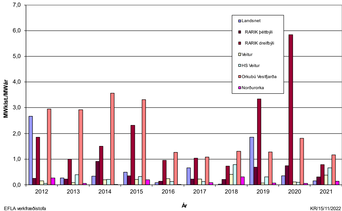
MYND 21 Stuðull um skerta orkuafhendingu, SSO, fyrir truflanir sem vara lengur en 3 mínútur árin 2012-2021.
