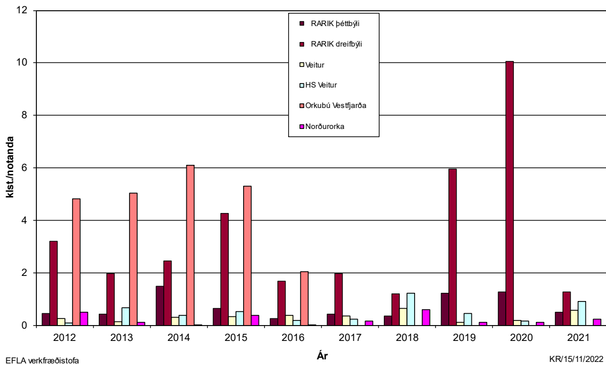
MYND 28 Stuðull um tímalengd straumleysis á hvern notanda, TSN (SAIDI), fyrir truflanatilvik sem vara lengur en 3 mínútur árin 2012-2021 (klst./notanda)
