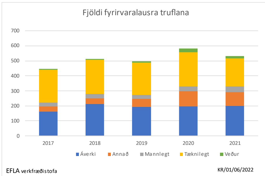
MYND 47 Fyrirvaralausar truflanir á lágspennu greindar eftir orsökum og árum.
