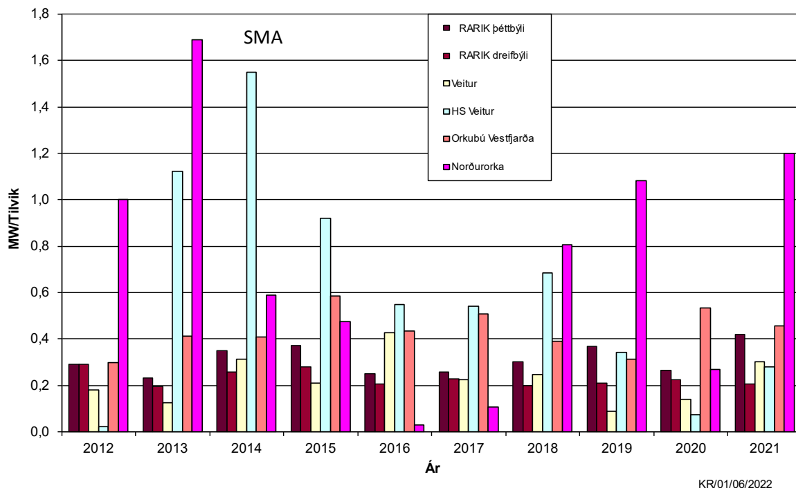
MYND 5 Stuðull um meðalskerðingu álags fyrir aðrar veitur en Landsnet, SMA, fyrir árin 2012-2021
