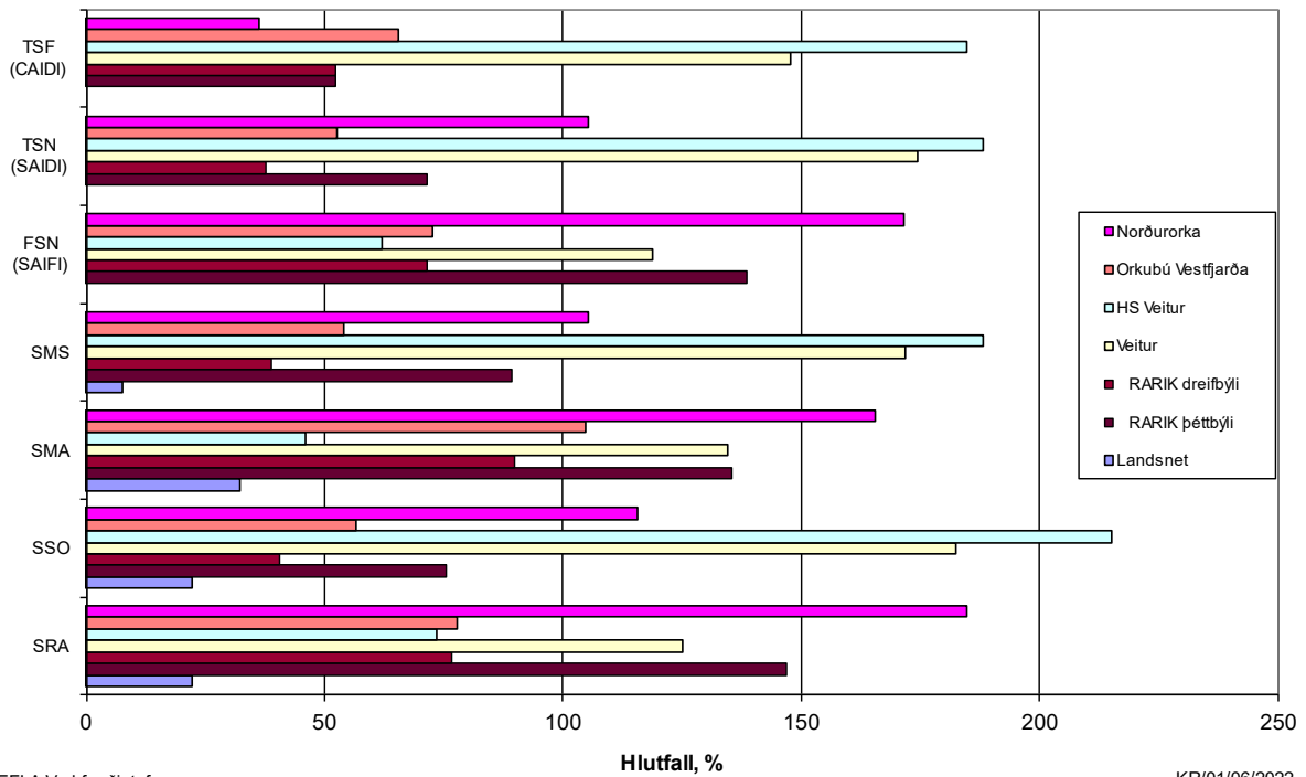
MYND 1 Samanburður á truflunum í raforkukerfi Landsnets og dreifiveitnanna árið 2021 við meðaltal árána 2012-2021 (árið 2021 í hlutfalli við meðaltalið)
