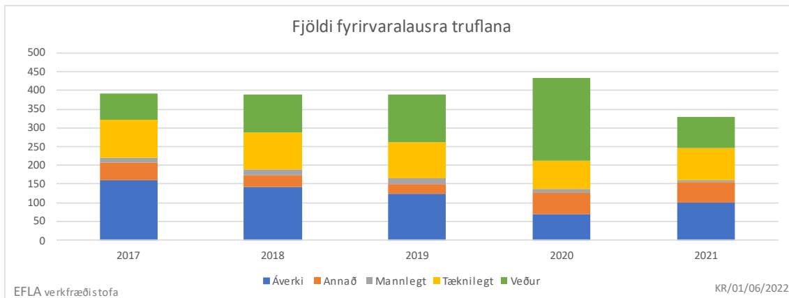
MYND 44 Fyrirvaralausar truflanir á háspennu greindar eftir orsökum og árum.
