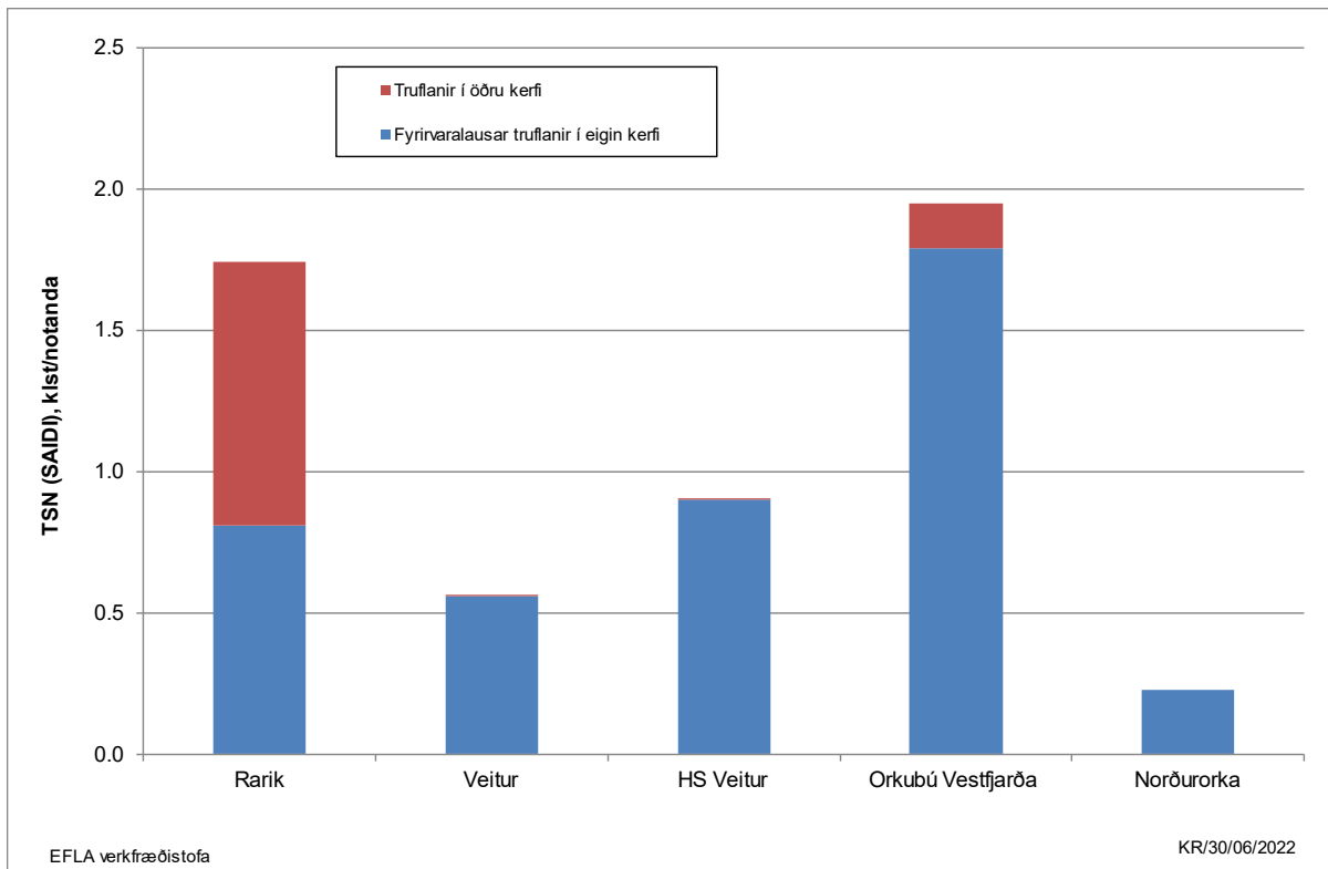
MYND 35 Stuðull um tímalengd straumleysis á hvern notanda, TSN (SAIDI) árið 2021 (kst./notanda).
