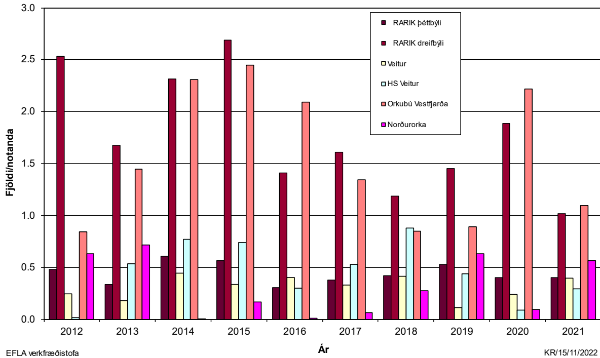
MYND 27 Stuðull um fjölda straumleysistilvika á hvern notanda, FSN (SAIFI), fyrir truflanatilvik sem vara lengur en 3 mínútur árin 2012-2021 (fjöldi/notanda).
