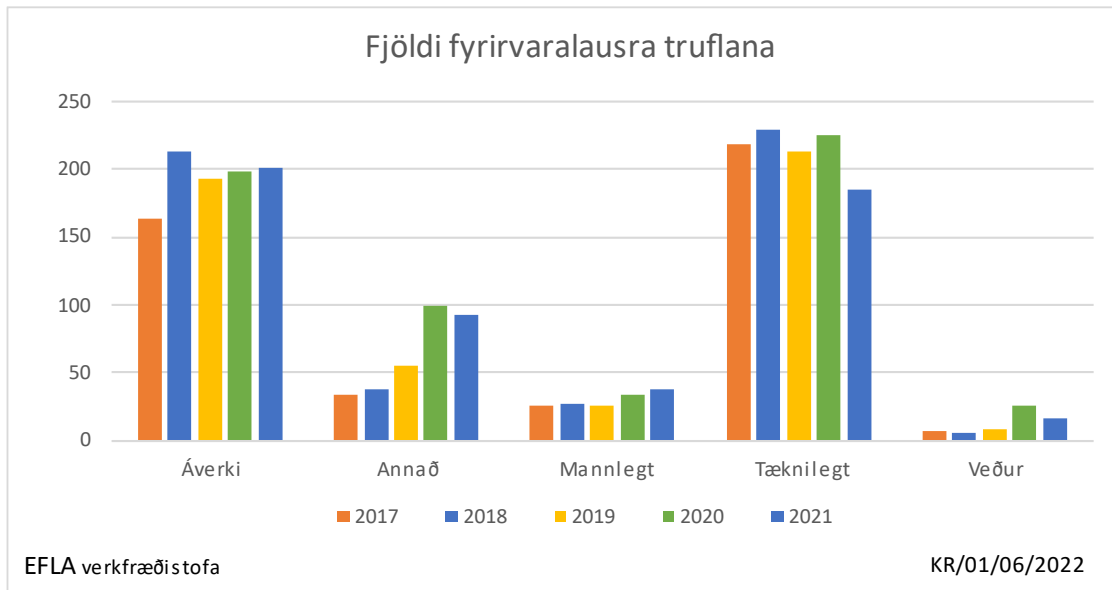
MYND 46 Fyrirvaralausar truflanir á lágspennu greindar eftir orsökum.
