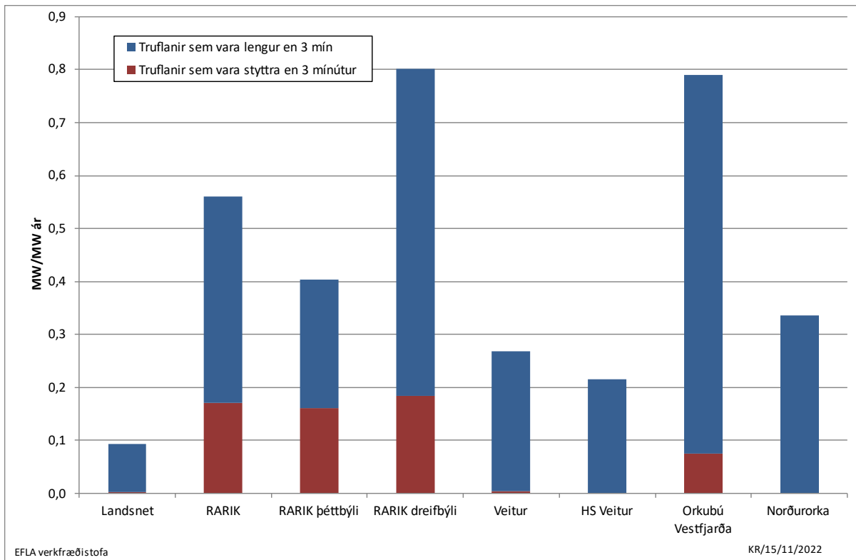
MYND 15 Stuðull um rofið álag, SRA, árið 2021 skipt eftir því hvort truflanirnar vara styttra eða lengur en 3 mín. (MW/MW-ár).
