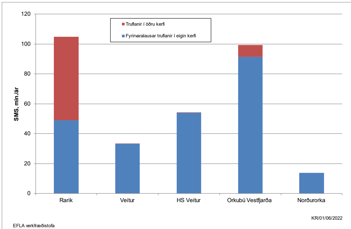
MYND 33 Stuðull um meðallengd skerðingar, SMS, árið 2021.
