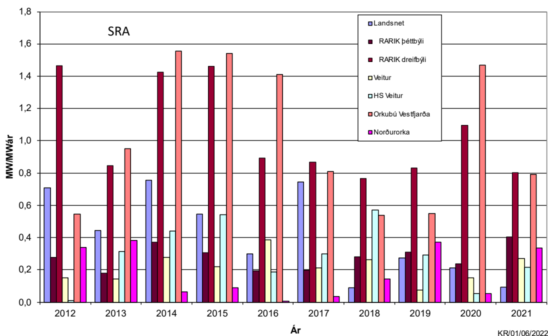
MYND 2 Stuðull um rofið álag, SRA, fyrir árin 2012-2021
