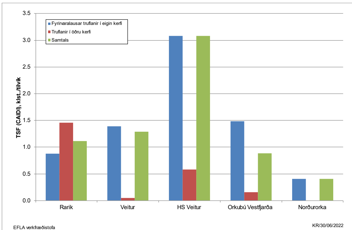
MYND 36 Stuðull um tímalengd straumleysis á hvert tilvik skerðingar, TSF (CAIDI), fyrir árið 2021 (kst./tilvik).
