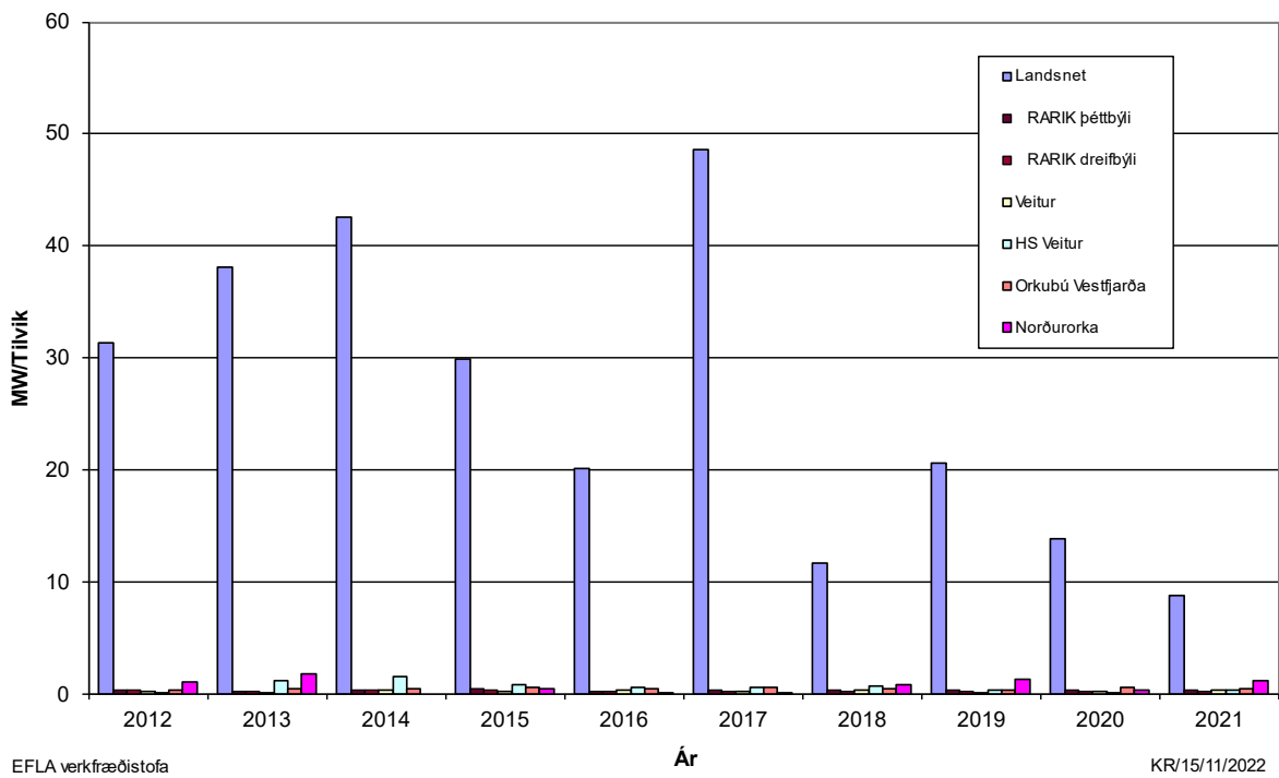
MYND 22 Stuðull um meðalskerðingu álags, SMA, fyrir truflanir sem vara lengur en 3 mínútur árin 2012-2021.
