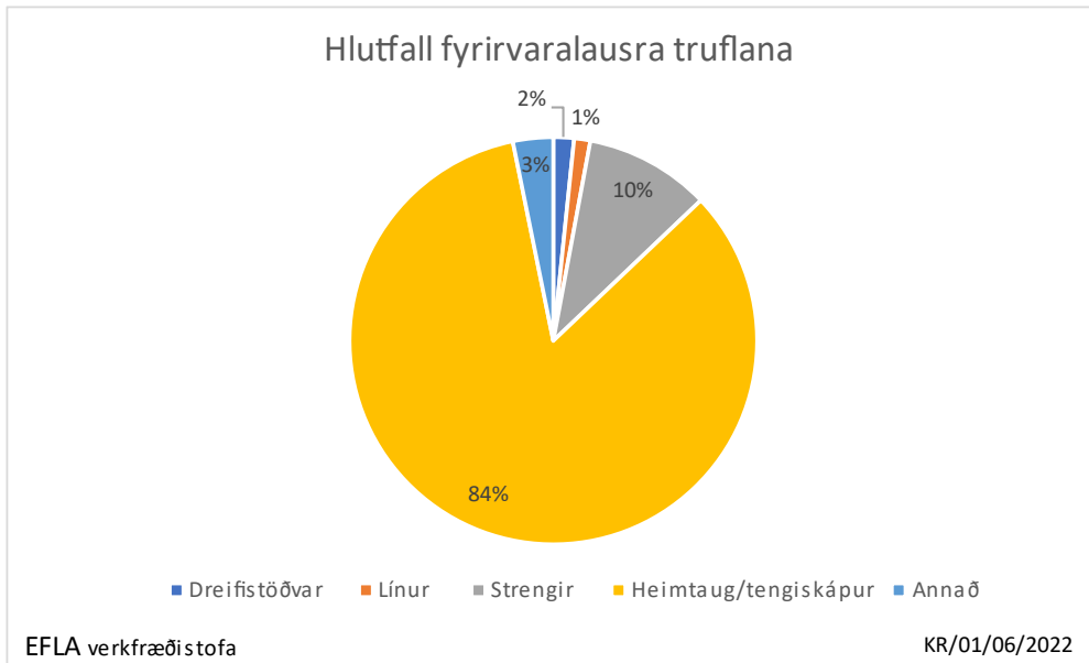
MYND 42 Hlutfall fyrirvaralausra truflana á lágspennu greindar eftir einingum 2017-2021
