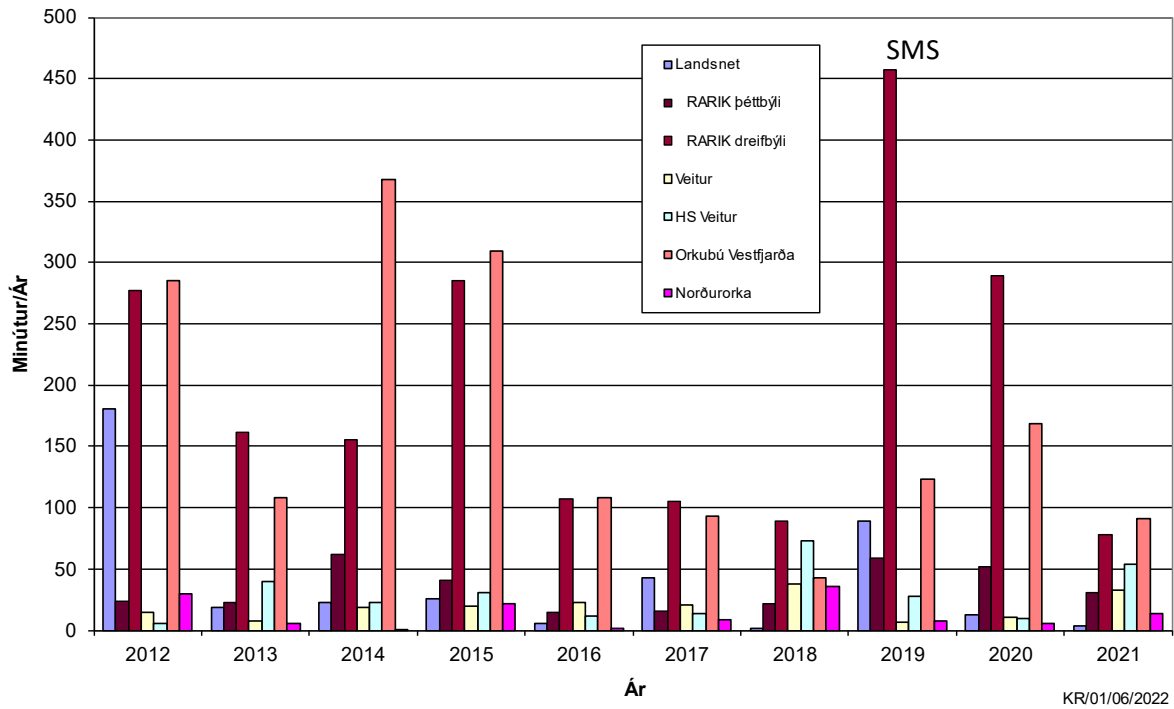
MYND 6 Stuðull um meðallengd skerðingar, oft nefnt straumleysismínútur, SMS, fyrir árin 2012-2021
