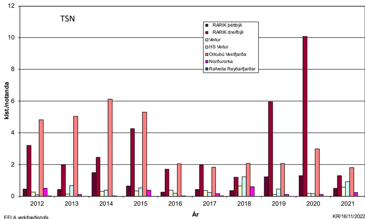
MYND 12 Stuðull um tímalengd straumleysis á hvern notanda, TSN (SAIDI), árin 2012-2021
