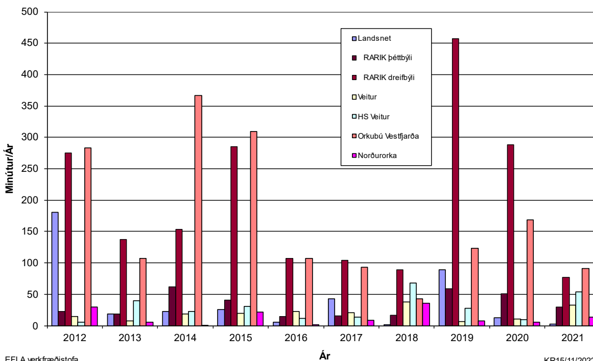
MYND 24 Stuðull um meðallengd skerðingar, SMS, fyrir truflanir sem vara lengur en 3 mínútur árin 2012-2021.
