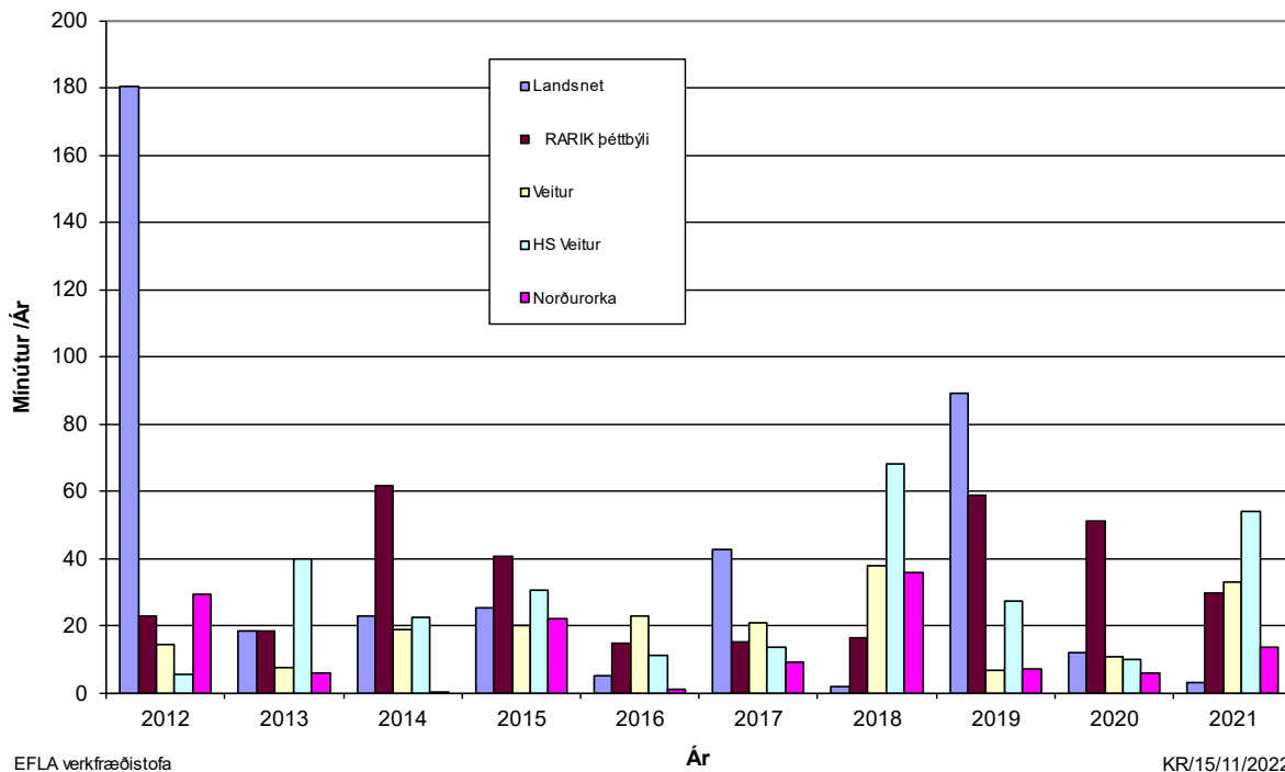
MYND 25 Stuðull um meðallengd skerðingar, SMS, fyrir truflanir sem vara lengur en 3 mínútur árin 2012-2021, þegar Orkubú Vestfjarða og RARIK dreifbýli hafa verið tekin úr myndinni.
