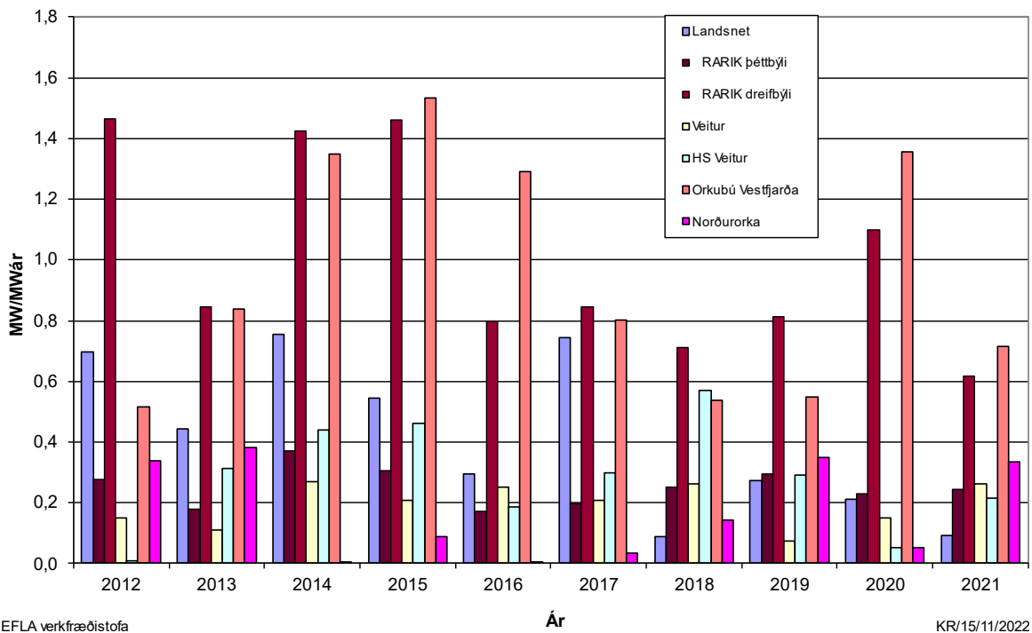
MYND 20 Stuðull um rofið álag, SRA, fyrir árin 2012-2021, fyrir truflanir sem vara lengur en 3 mínútur.
