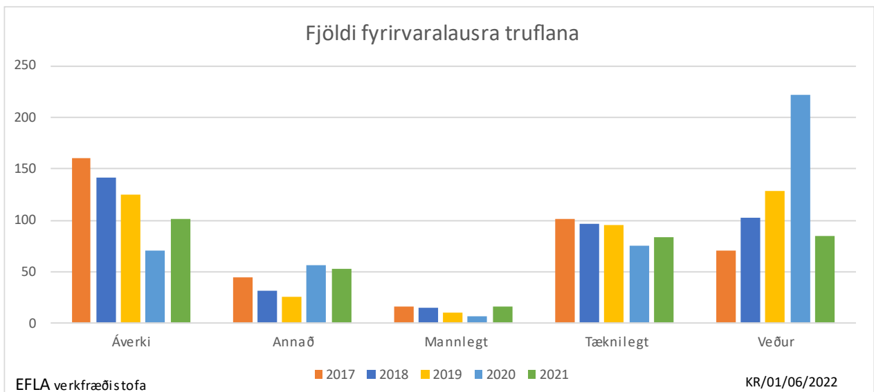
MYND 43 Fyrirvaralausra truflanir á háspennu greindar eftir orsökum.
