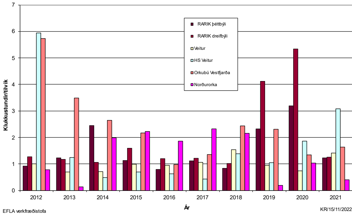
MYND 29 Stuðull um tímalengd straumleysis á hvert tilvik skerðingar, TSF (CAIDI), fyrir truflanatilvik sem vara lengur en 3 mínútur árin 2012-2021 (klst./tilvik)
