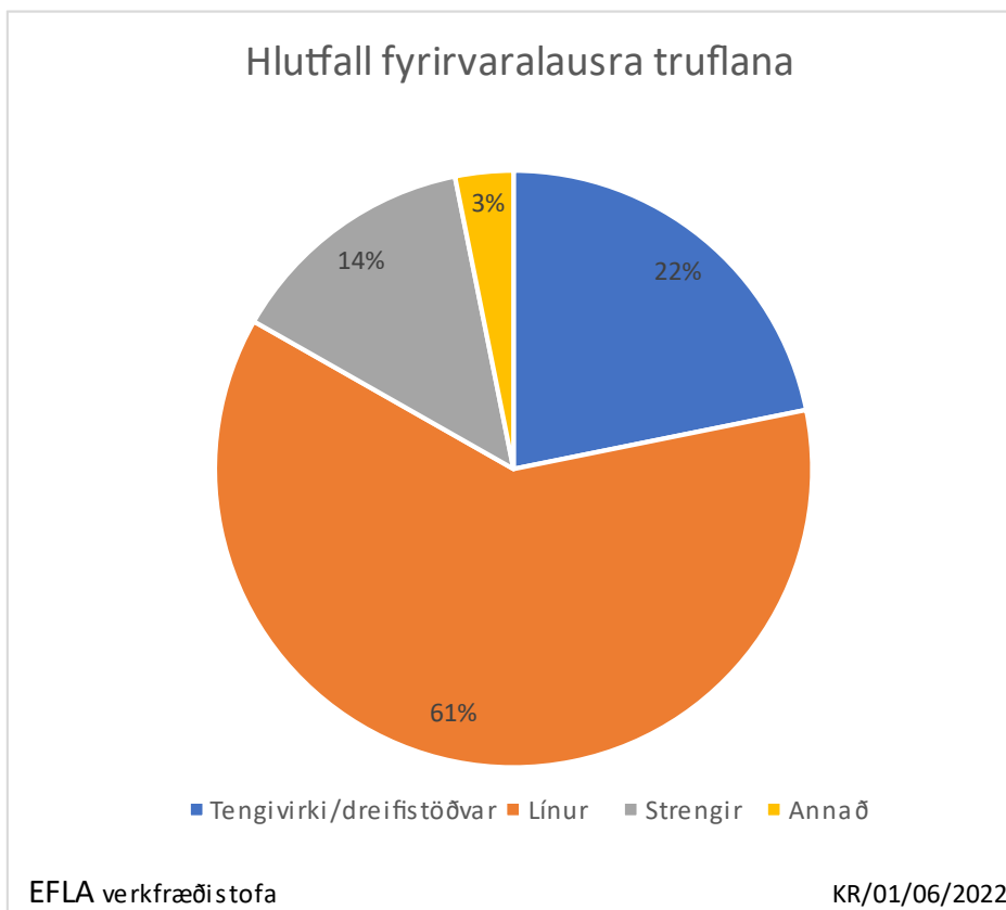
MYND 39 Hlutfall fyrirvaralausar truflanir á háspennu greindar eftir einingum 2017-2021
