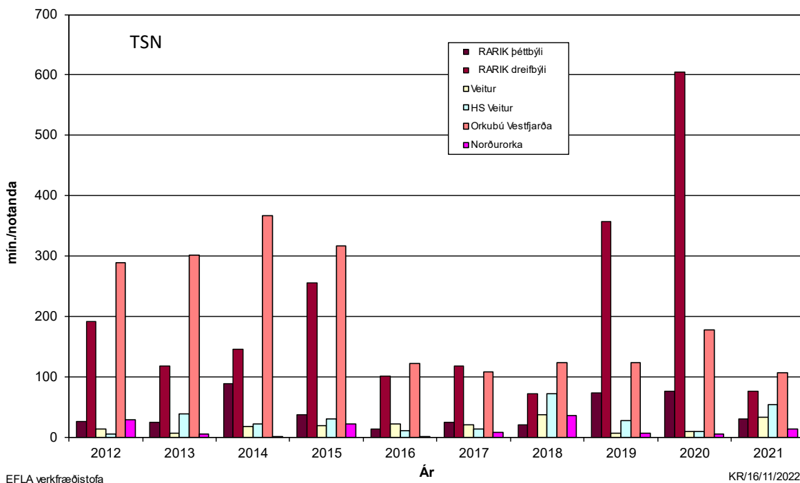
MYND 13 Stuðull um tímalengd straumleysis á hvern notanda, TSN (SAIDI), árin 2012-2021 í mínútum á notanda.
