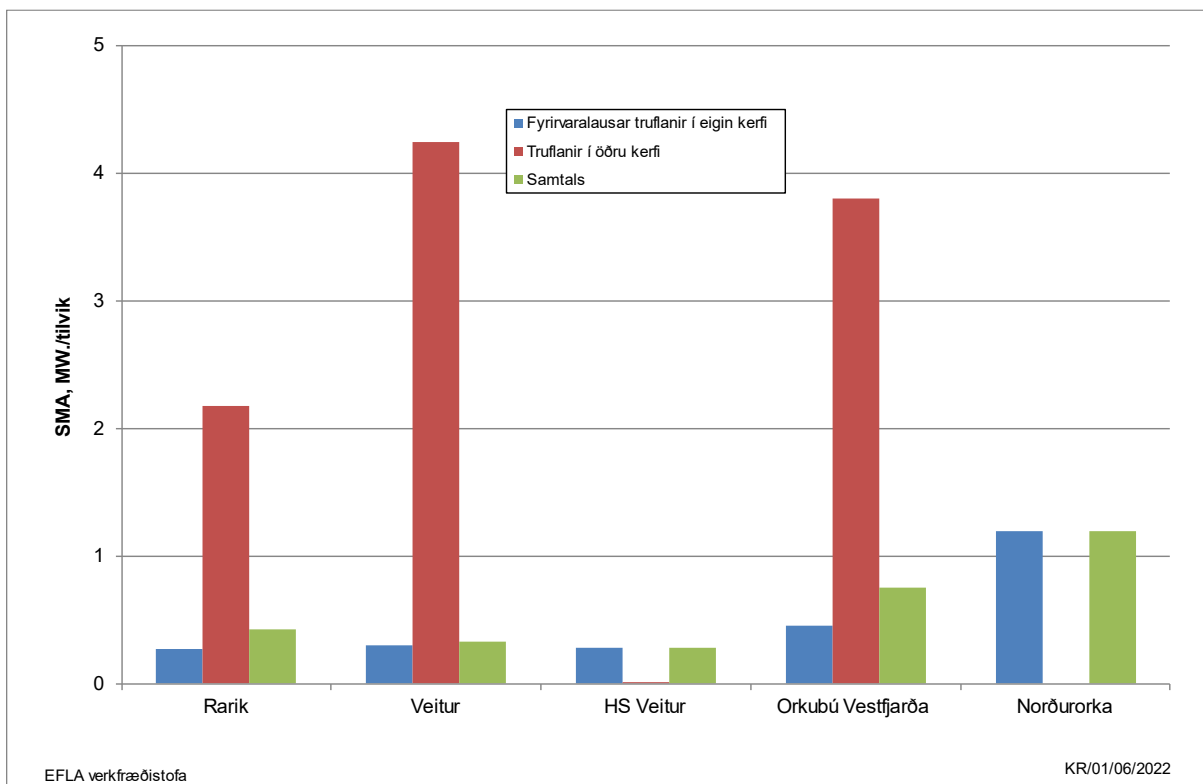
MYND 32 Stuðull um meðalskerðingu álags, SMA, fyrir árið 2021.
