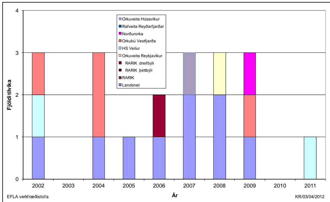
Mynd 9 Fjöldi skerðingartilvika árin 2002-2011 sem eru á bilinu 10 til 100 kerfismínútur.
