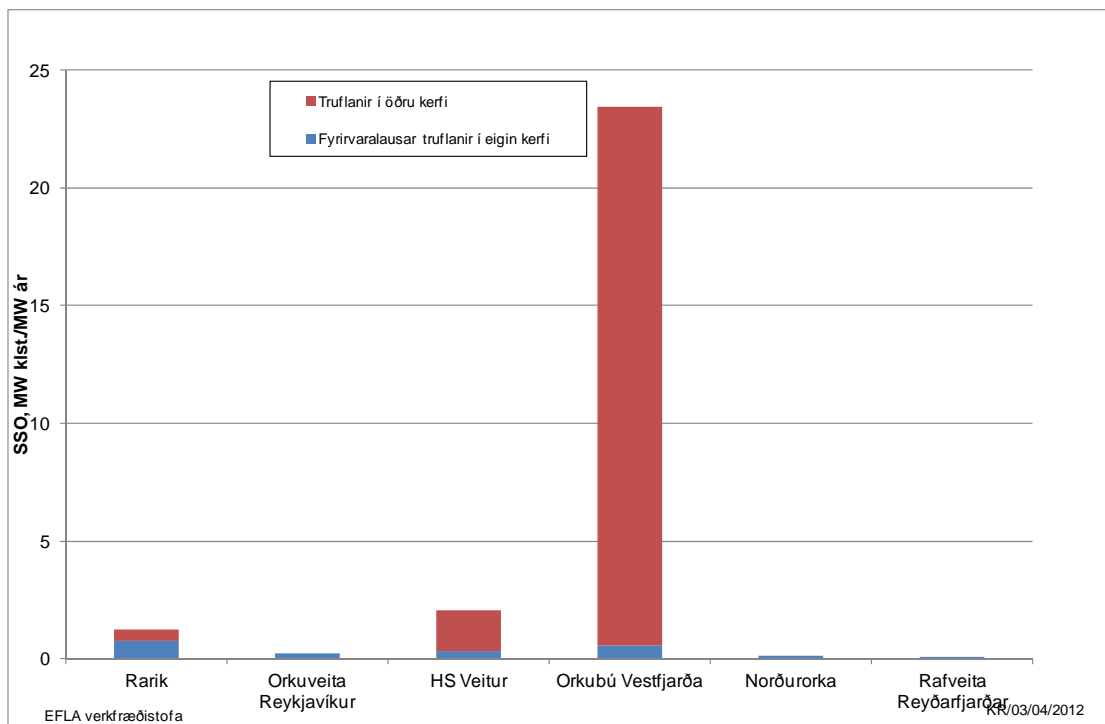
Mynd 20 Stuðull um skerta orkuafhendingu, SSO, árið 2011.
