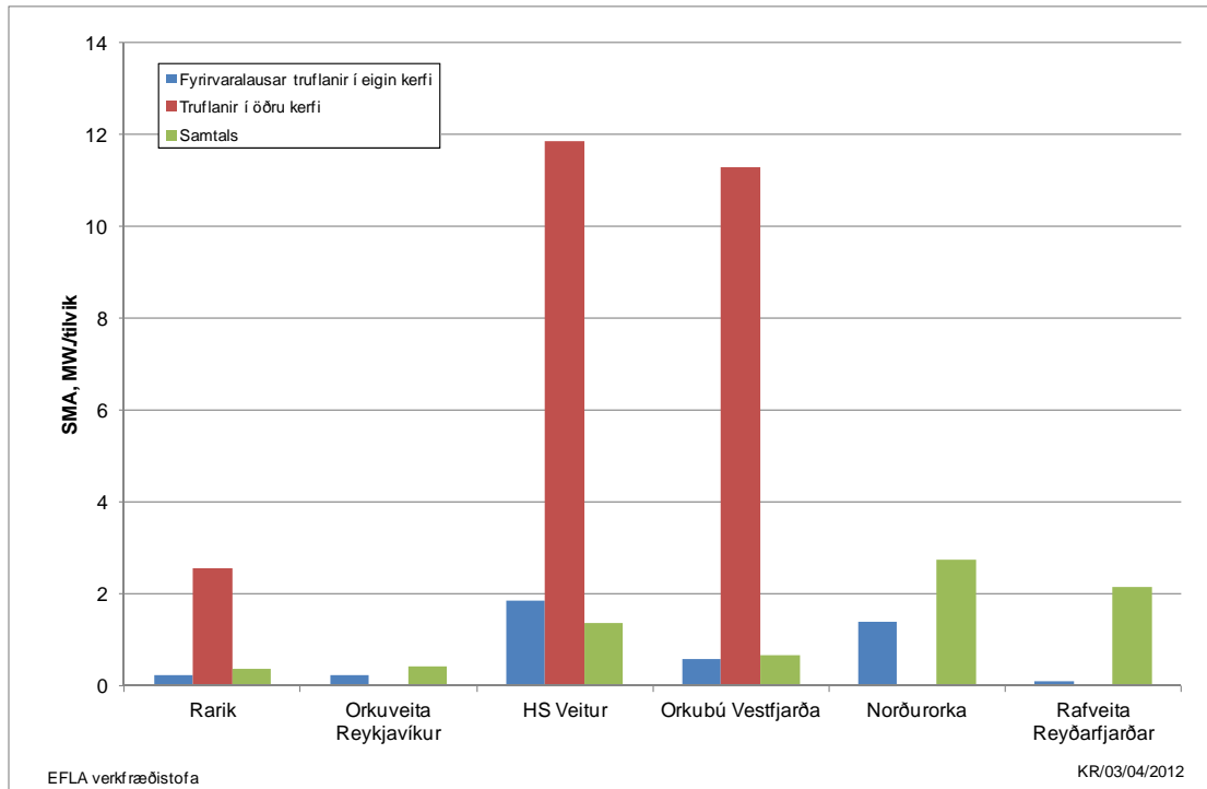
Mynd 21 Stuðull um meðalskerðingu álags, SMA, árið 2011.
