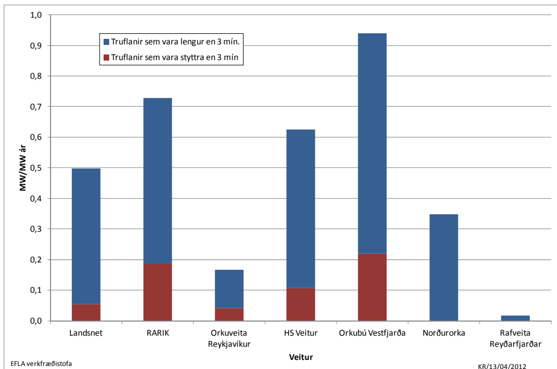
Mynd 14 Stuðull um rofið álag, SRA, árið 2011 skipt eftir því hvort truflanirnar vara styttra eða lengur en 3 mín.
