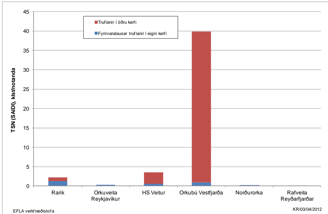
Mynd 25 Stuðull um tímalengd straumleysis á hvern notanda, TSN (SAIDI), árið 2011.
