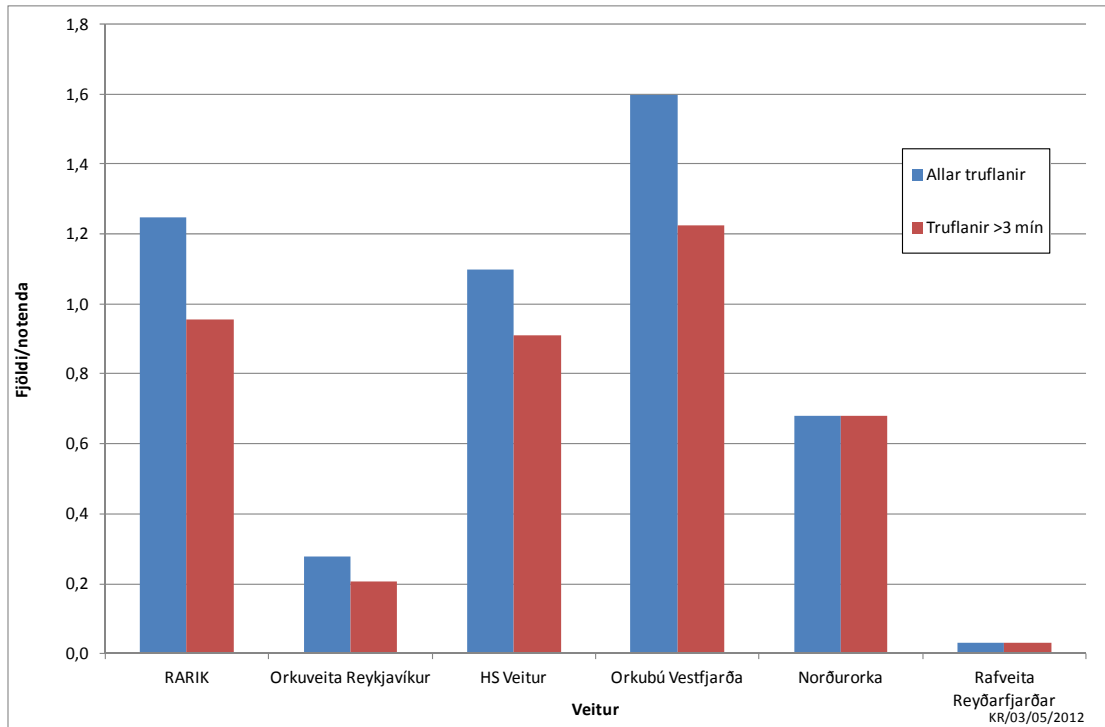
Mynd 16 Stuðull um fjölda straumleysistilvika á hvern notanda, FSN (SAIFI), árið 2011 fyrir allar truflanir og truflanir sem vara lengur en 3 mín .
