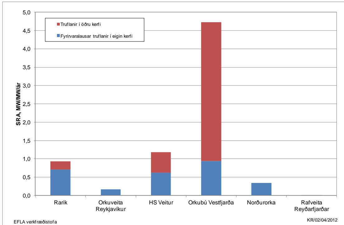
Mynd 19 Stuðull um rofið álag, SRA, árið 2011.
