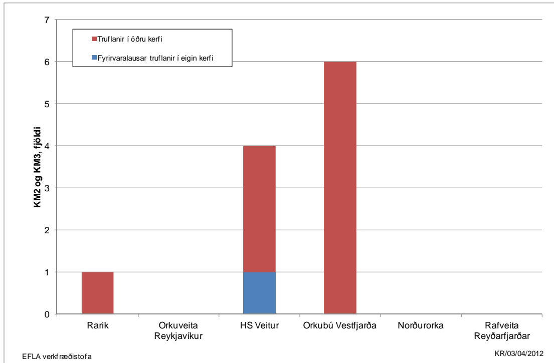
Mynd 23 Fjöldi skerðingartilvika árið 2011 sem eru meira en 10 kerfismínútur.
