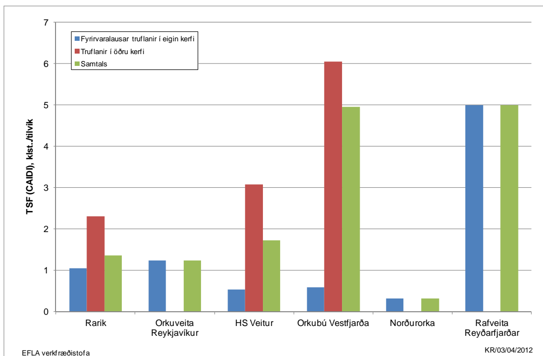
Mynd 26 Stuðull um tímalengd straumleysis á hvert tilvik skerðingar, TFSF (CAIDI), árið 2011 (klst./tilvik).
