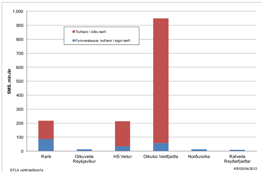
Mynd 22 Stuðull um meðallengd skerðingar, SMS, árið 2011.
