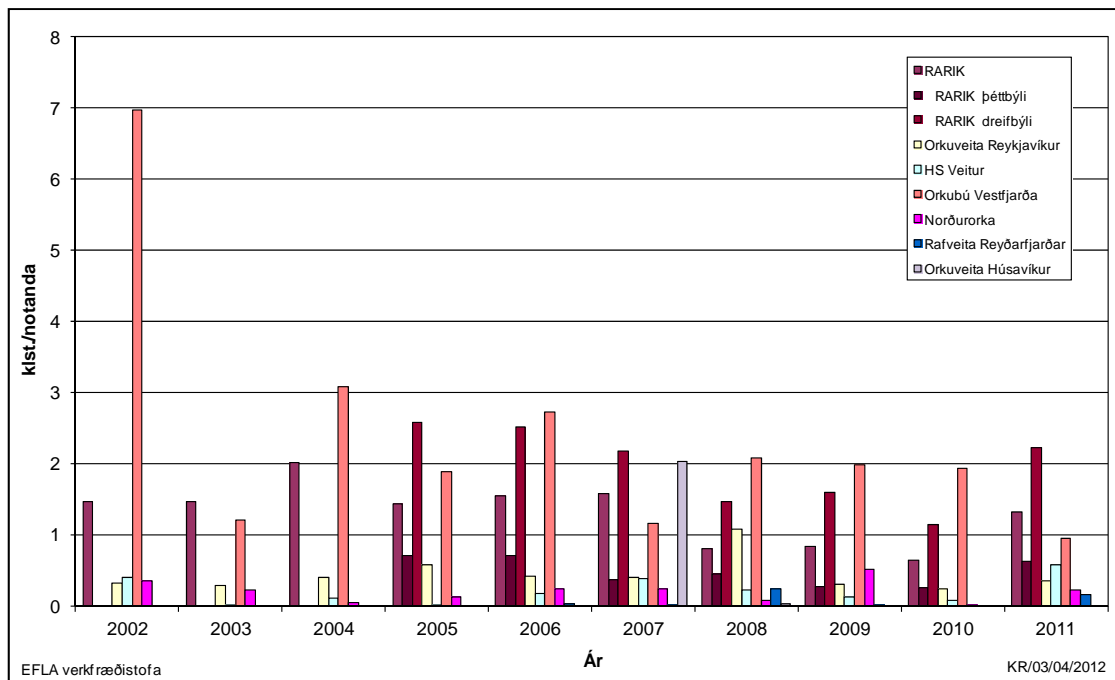
Mynd 12 Stuðull um tímalengd straumleysis á hvern notanda, TSN (SAIDI), árin 2002-2011 .
