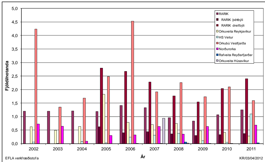
Mynd 11 Stuðull um fjölda straumleysistilvika á hvern notanda, FSN (SAIFI), árin 2002-2011 .
