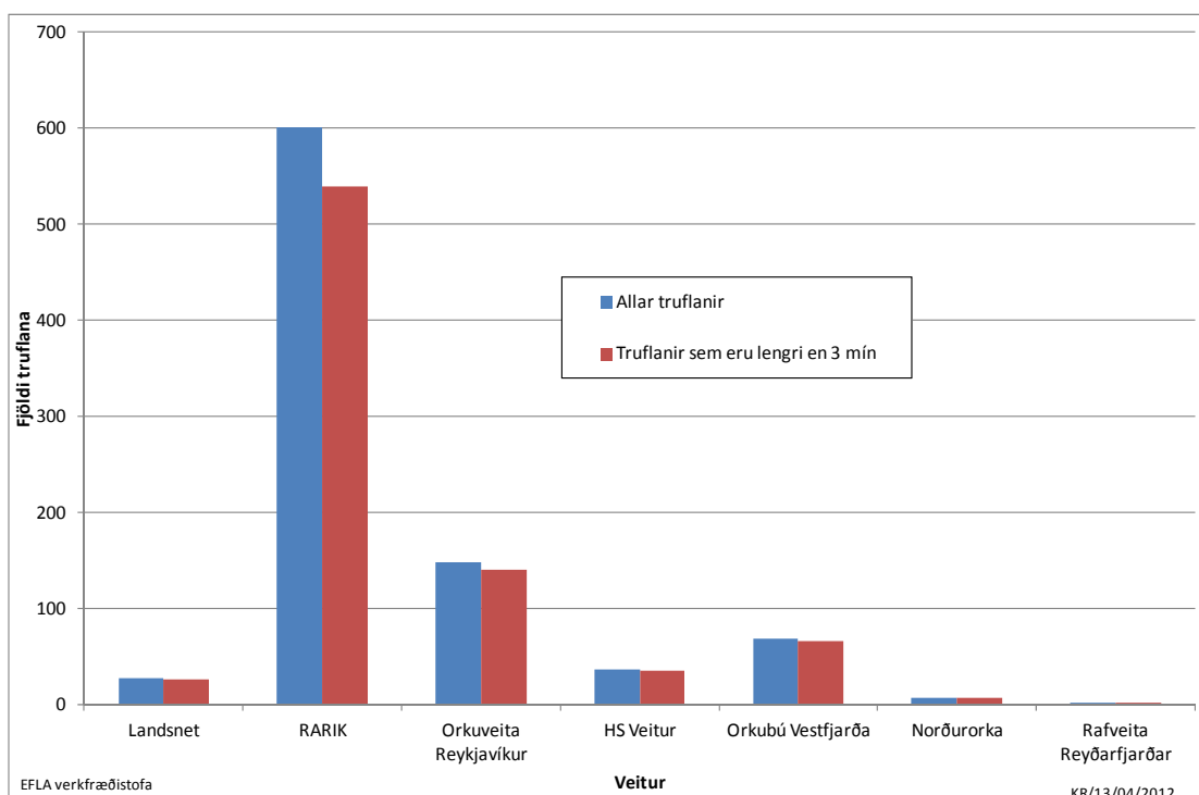
Mynd 15 Heildarfjöldi skerðingartilvika árið 2011, sýndar eru annars vegar allar truflanir og hins vegar truflanir sem vara lengur en 3 mínútur.
