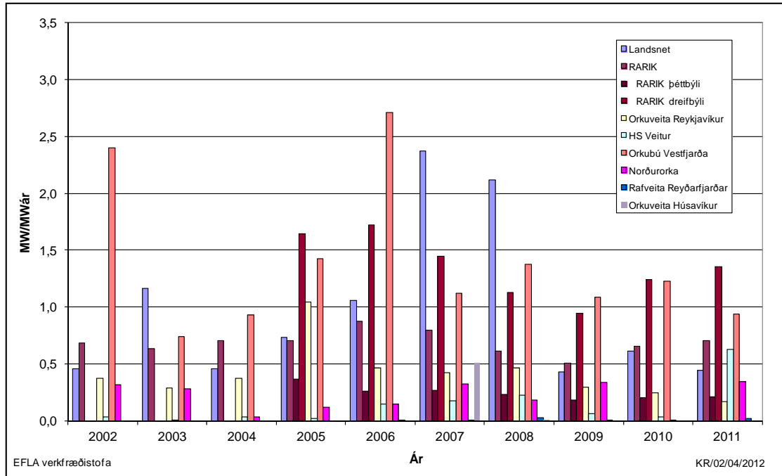
Mynd 1 Stuðull um rofið álag, SRA, árin 2002-2011 .
