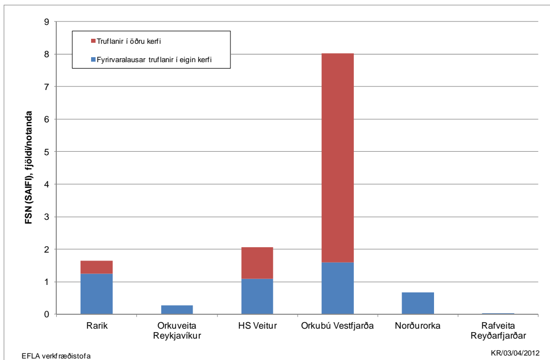
Mynd 24 Stuðull um fjölda straumleysistilvika á hvern notanda, FSN (SAIFI), árið 2011.
