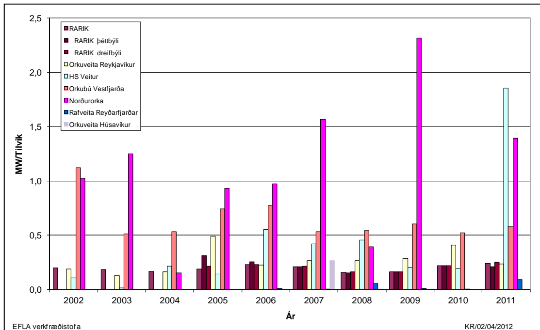
Mynd 4 Stuðull um meðalskerðingu álags, SMA, fyrir aðrar veitur en Landsnet árin 2002-2011 .
