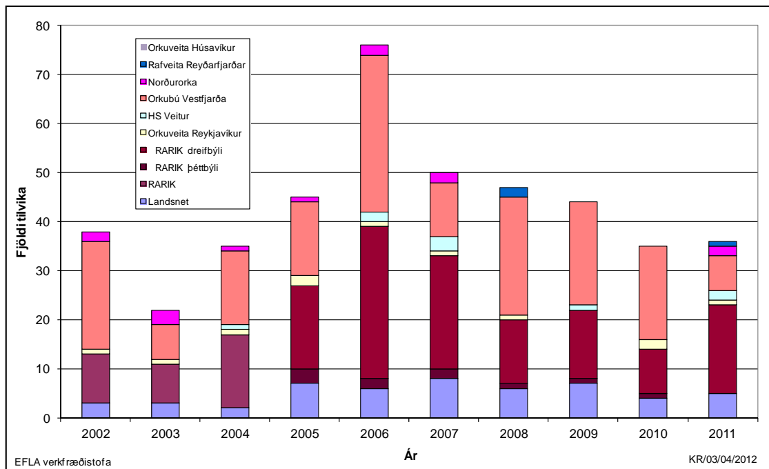
Mynd 8 Fjöldi skerðingartilvika árin 2002-2011 sem eru á bilinu 1 til 10 kerfismínútur.
