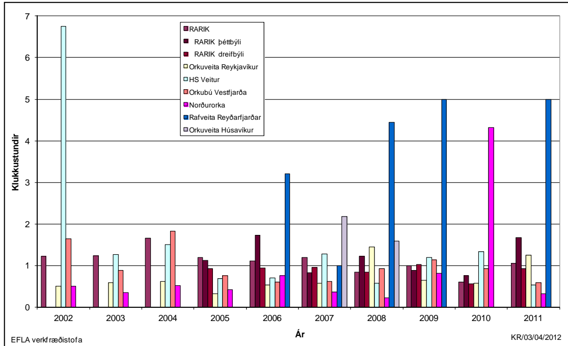
Mynd 13 Stuðull um tímalengd straumleysis á hvert tilvik skerðingar, TSF (CAIDI), árin 2002-2011 (klst/tilvik).
