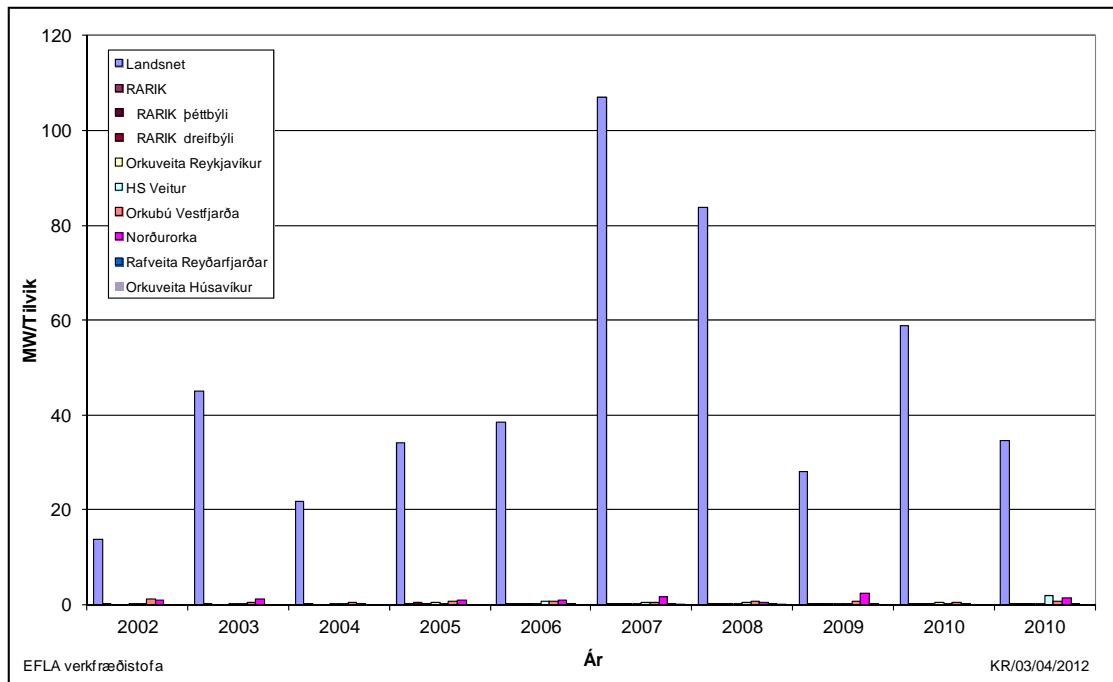
Mynd 3 Stuðull um meðalskerðingu álags, SMA, 2002-2011 .
