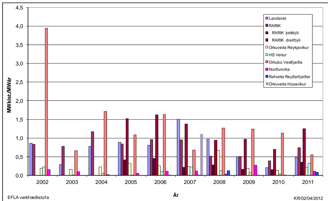
Mynd 2 Stuðull um skerta orkuafhendingu, SSO, árin 2002-2011 .
