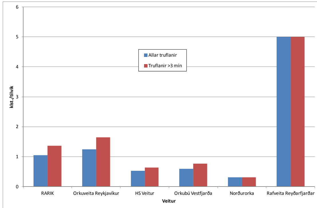
Mynd 18 Stuðull um tímalengd straumleysis á hvert tilvik skerðingar, TSF (CAIDI), árið 2011 fyrir allar truflanir og truflanir sem vara lengur en 3 mín
