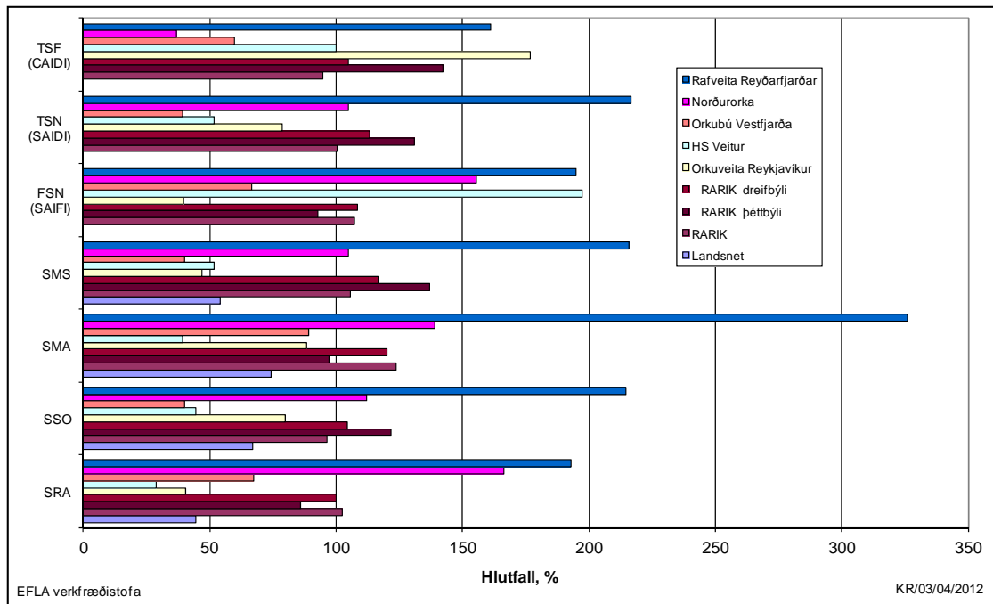
Mynd I Samanburður á truflunum í raforkukerfi Landsnets og stærstu dreifiveitnanna árið 2011 við meðaltal árána 2002-2011 (árið 2011 í hlutfalli við meðaltalið).
