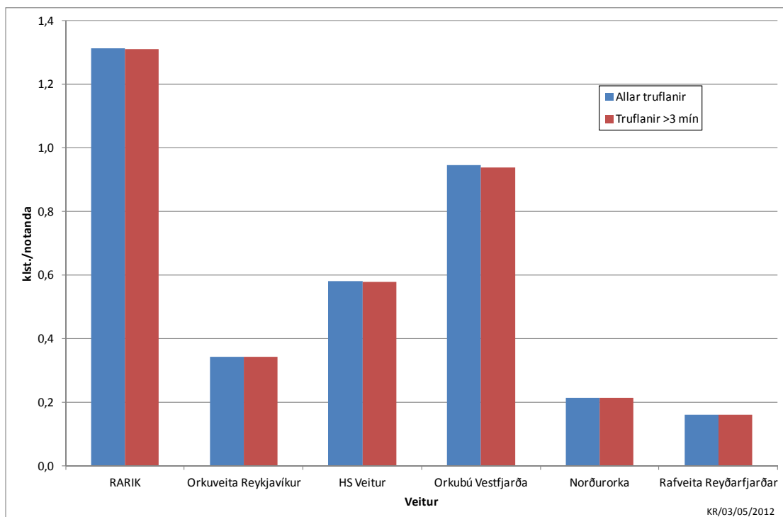
Mynd 17 Stuðull um tímalengd straumleysis á hvern notanda, TSN (SAIDI), árið 2011 fyrir allar truflanir og truflanir sem vara lengur en 3 mín .
