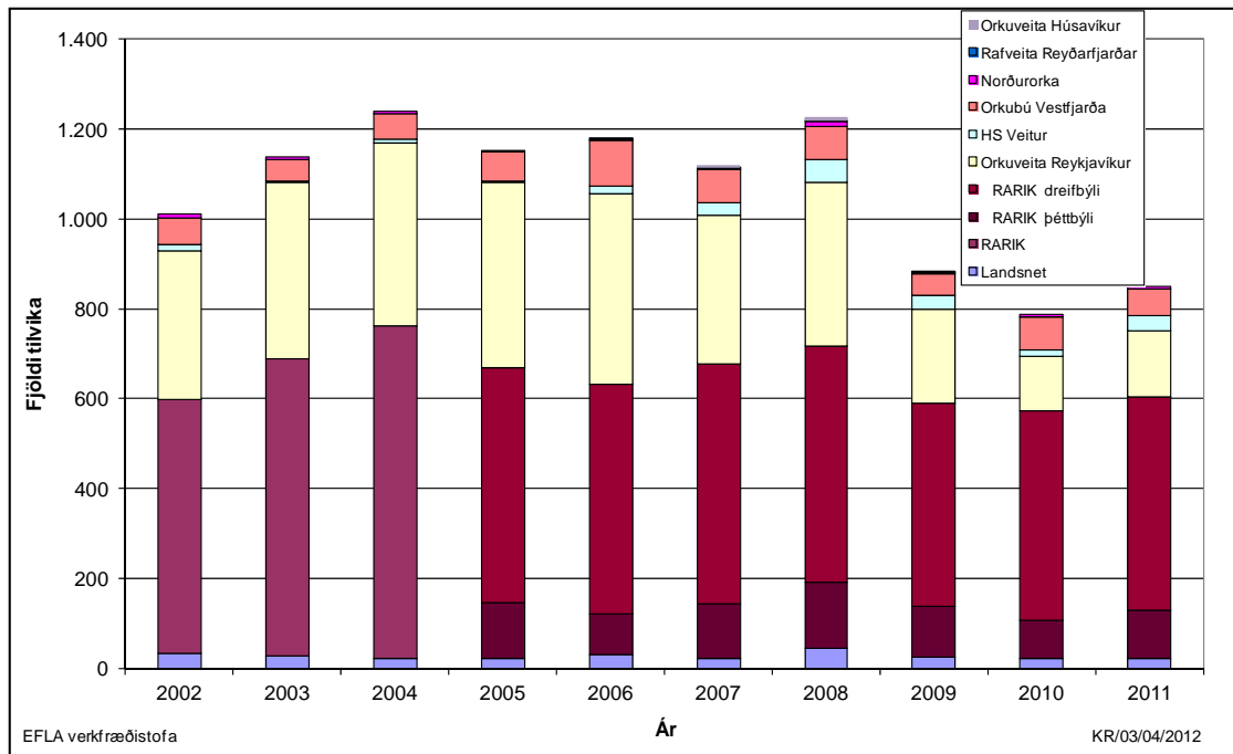
Mynd 7 Fjöldi skerðingartilvika árin 2002-2011 sem eru innan við 1 kerfismínúta.
