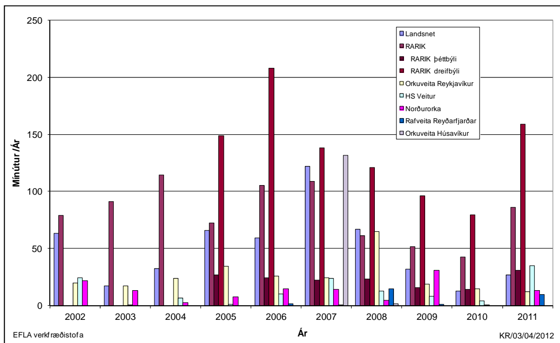
Mynd 6 Stuðull um meðallengd skerðingar, SMS, fyrir aðrar veitur en Orkubú Vestfjarða árin 2002-2011 .
